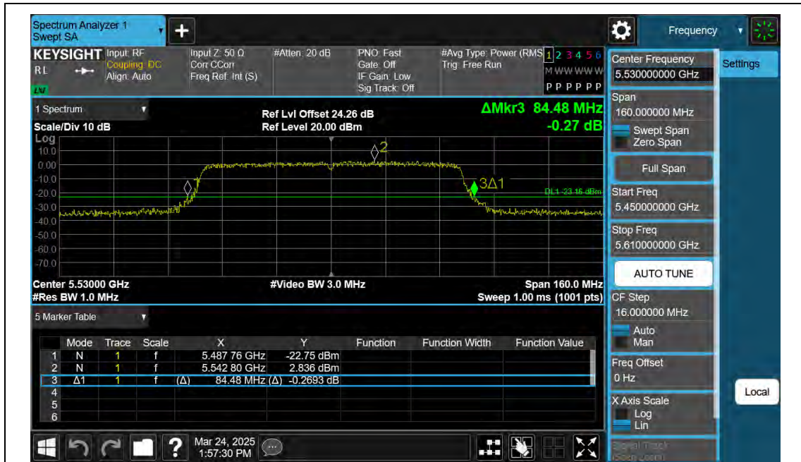
11AC80SISO-Ant2-5530
