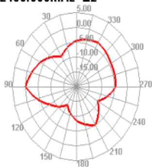
2450.000MHz E2
