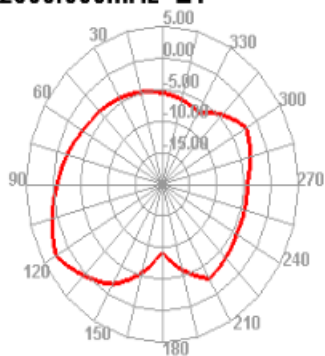
2500.000MHz E1
