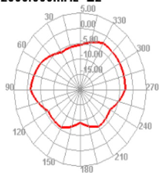
2500.000MHz E2
