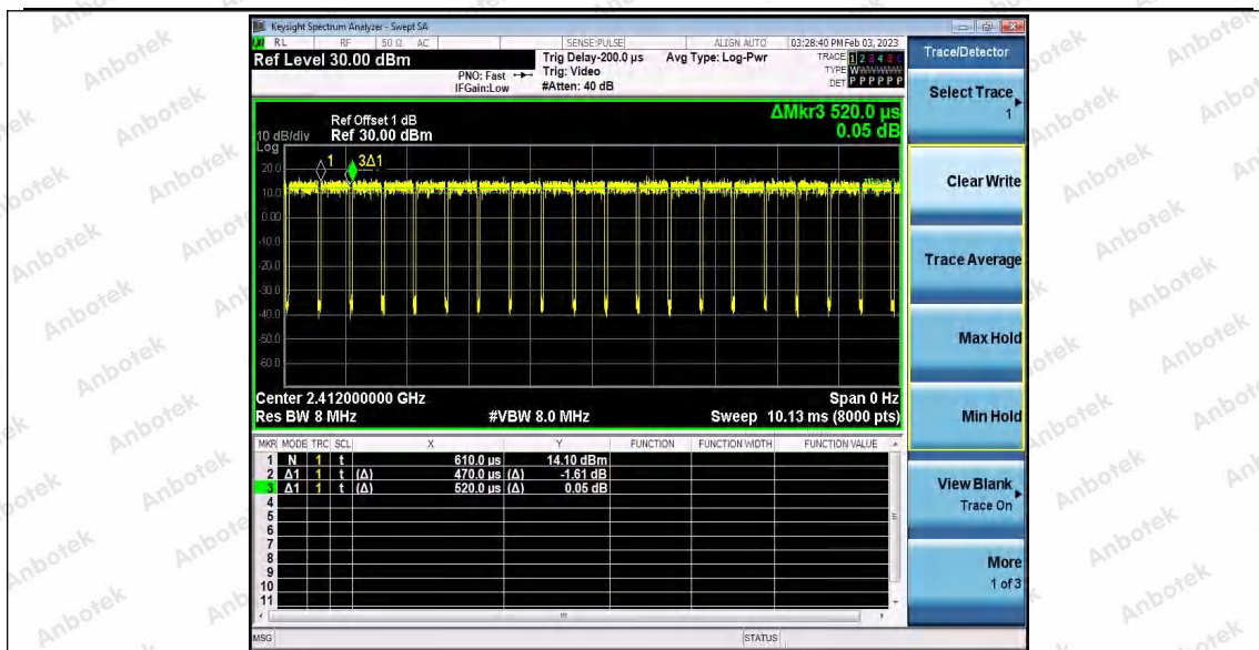
11N20_Ant2_2412
