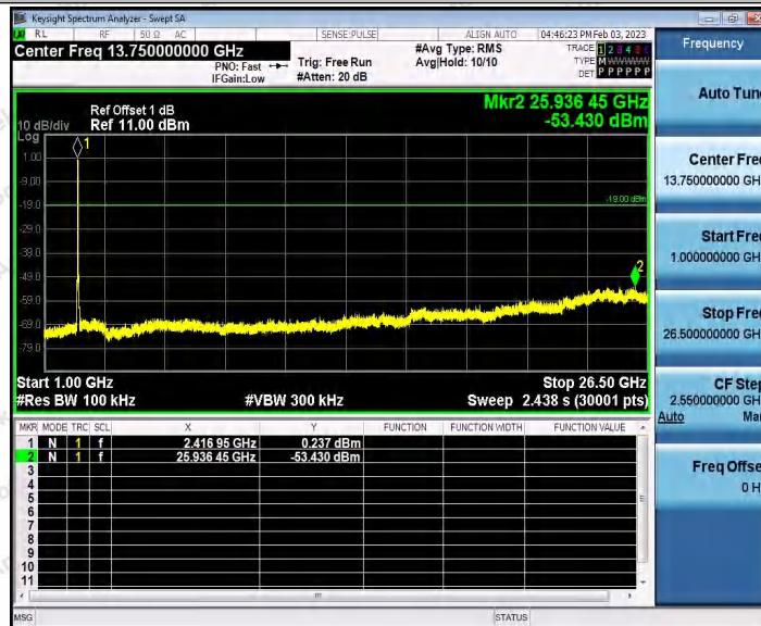
11N40_Ant1_2437_0~Reference
