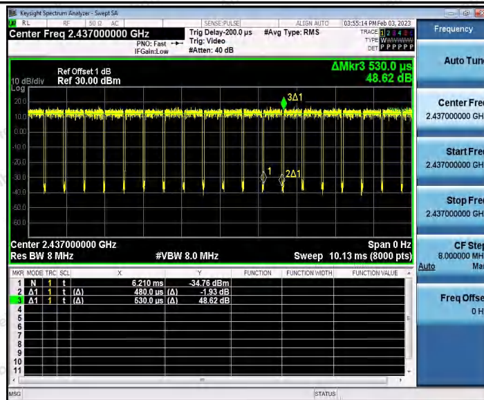
11AX20_Ant2_2437
