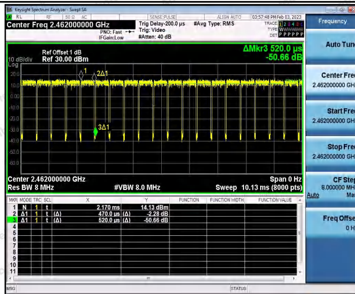
11AX20_Ant2_2462
