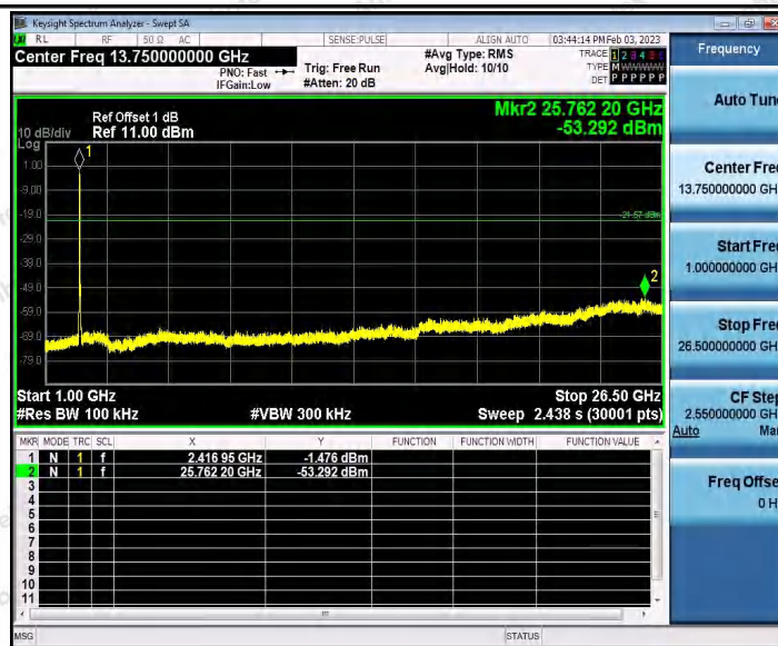
11N40_Ant2_2422_0~Reference
