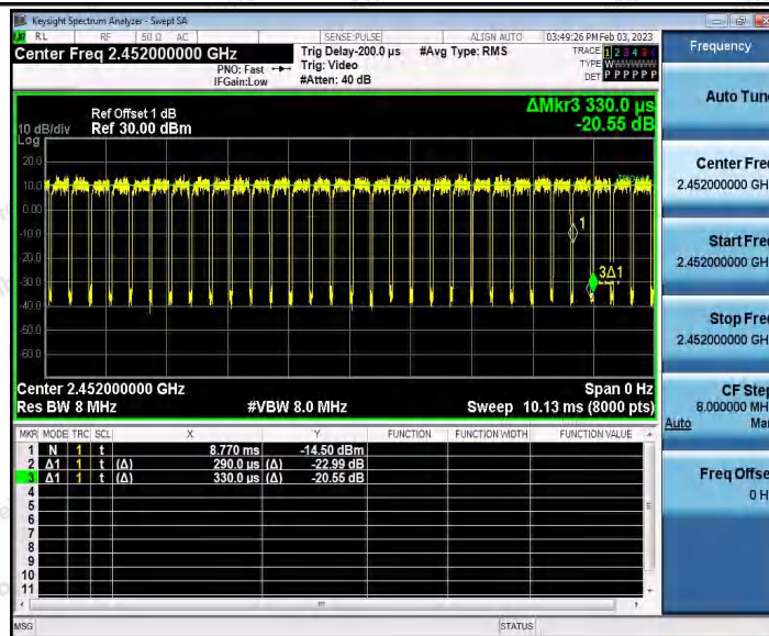
11N40_Ant2_2452
