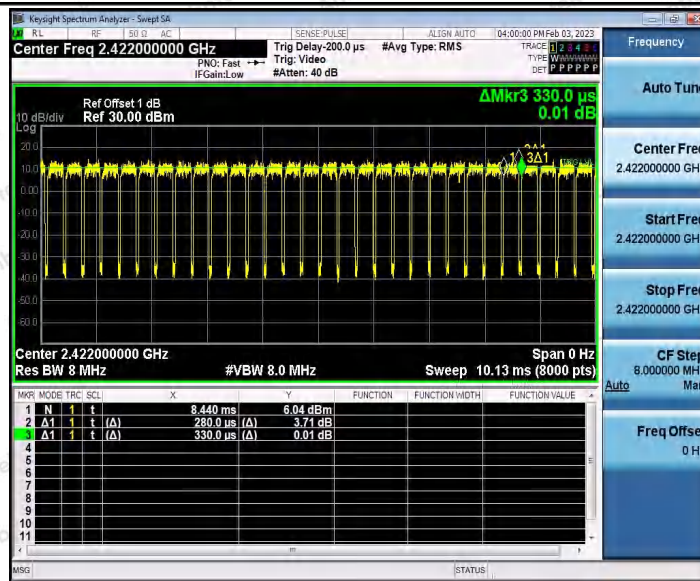
11AX40_Ant2_2422
