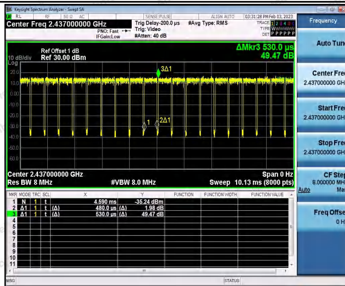
11N20_Ant2_2437
