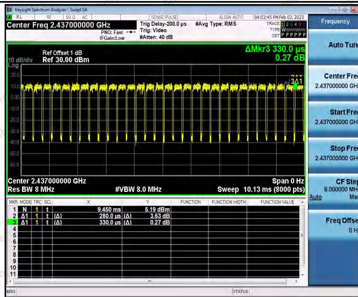
11AX40_Ant2_2437
