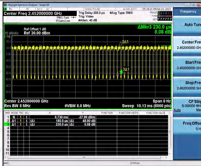
11AX40_Ant2_2452
