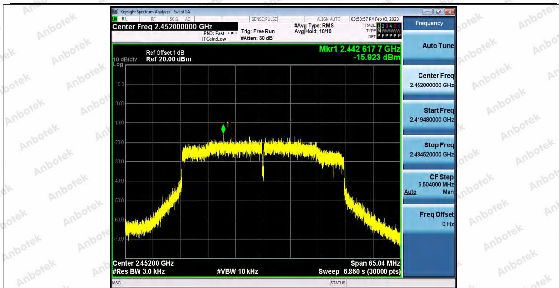
11N40_Ant2_2452
