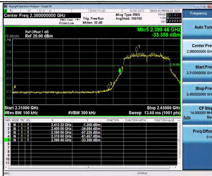
11AX40_Ant2_Low_2422
