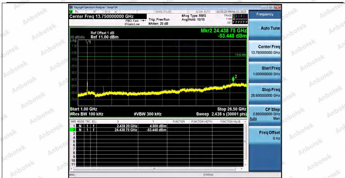
11B_Ant2_2437_0~Reference
