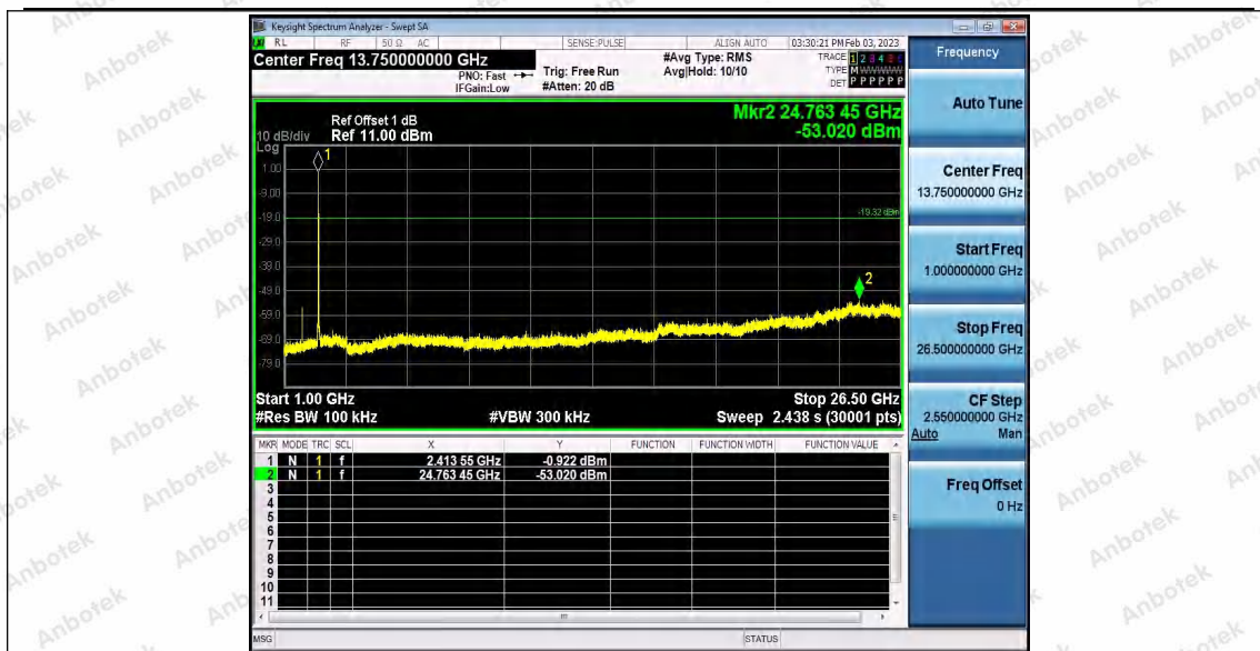
11N20_Ant2_2412_0~Reference
