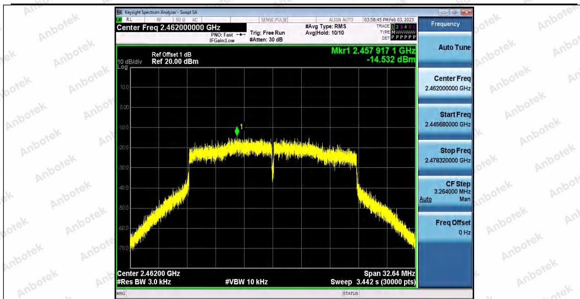
11AX20_Ant2_2462
