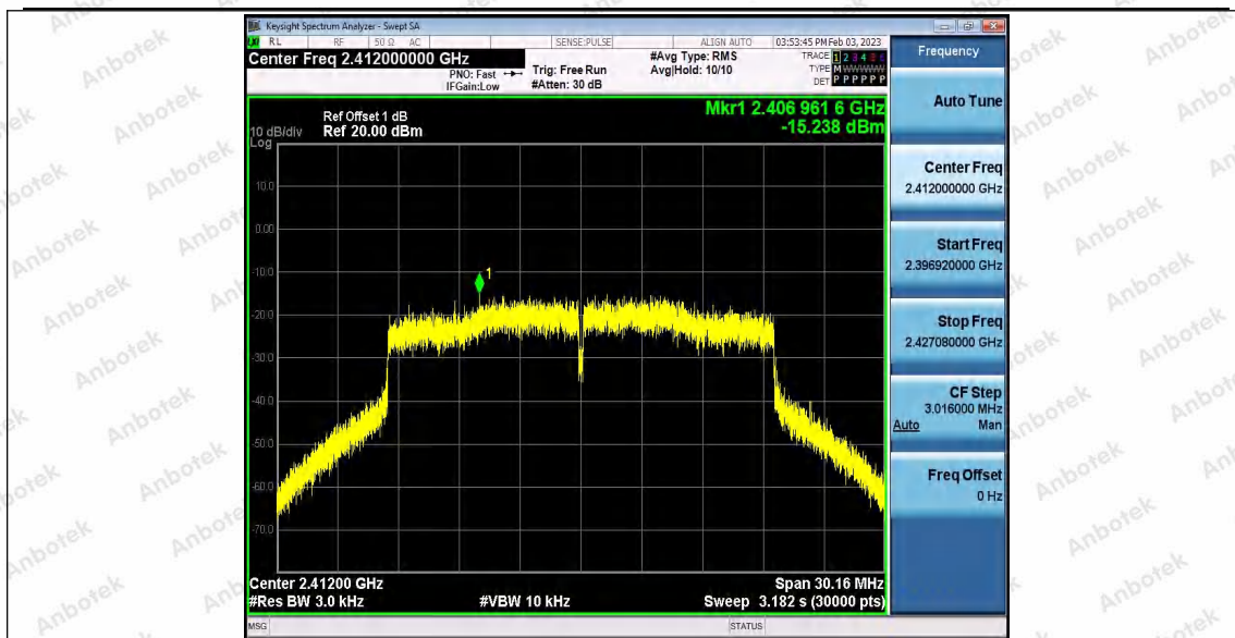
11AX20_Ant2_2412
