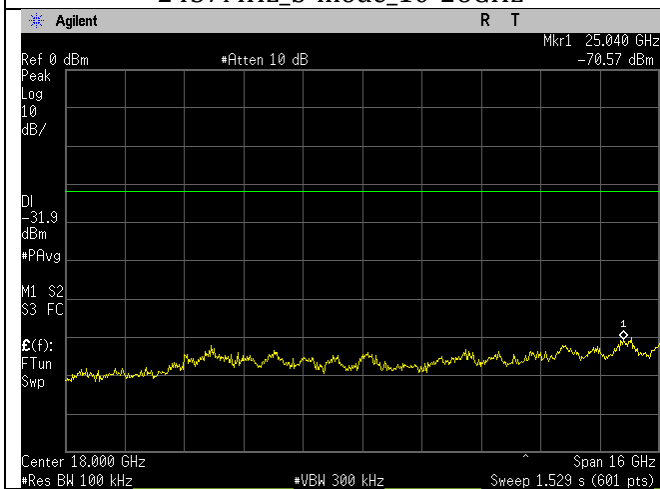
2437MHz_g-mode_10-26GHz
