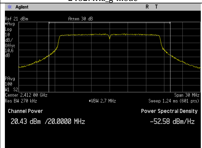
2412MHz_g-mode
