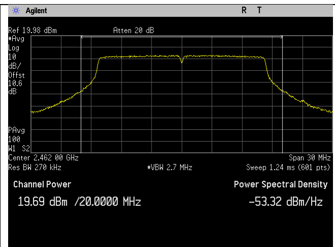
2462MHz_g-mode
