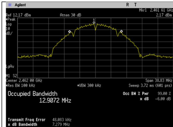
2462MHz_b-mode_-6dB
