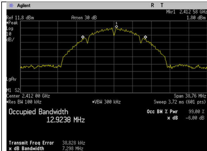
2412MHz_b-mode_-6dB
