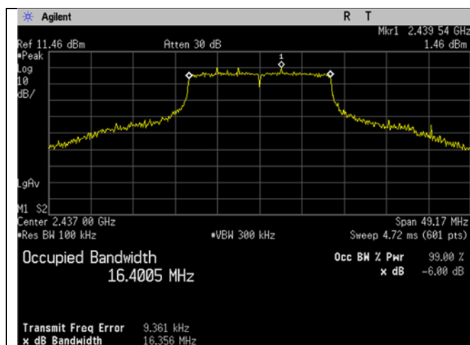
2437MHz_g-mode_-6dB
