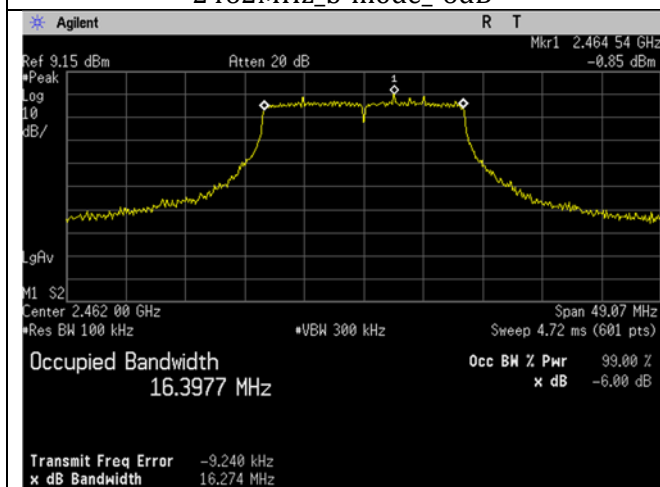
2462MHz_g-mode_-6dB
