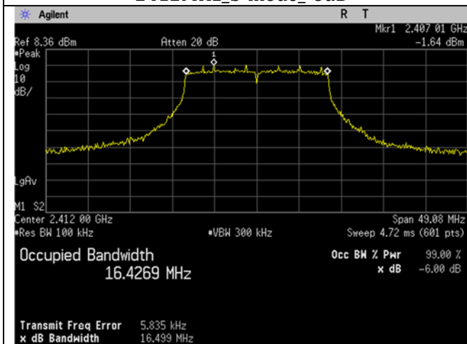
2412MHz_g-mode_-6dB
