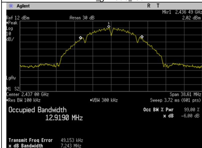
2437MHz_b-mode_-6dB
