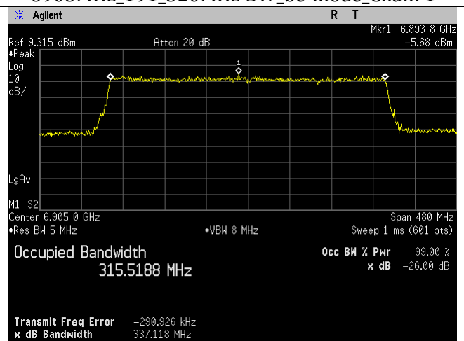
6905MHz_191_320MHz BW_be-mode_Chain 3
