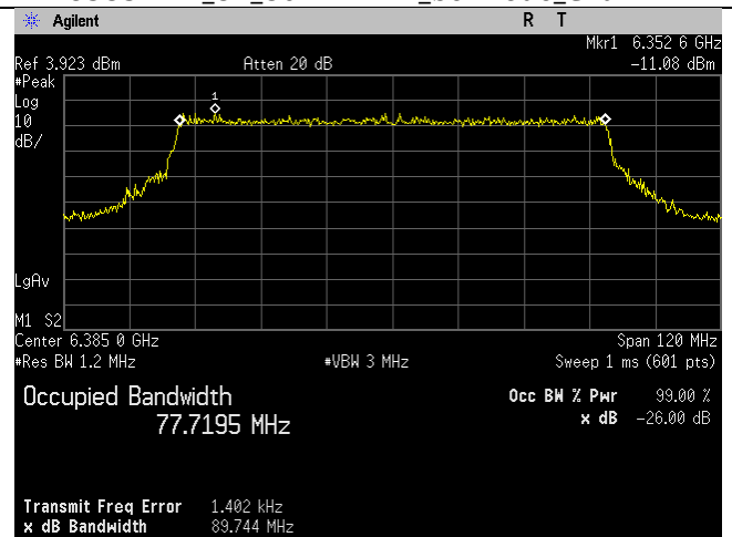
6385MHz_87_80MHz BW_be-mode_Chain 3
