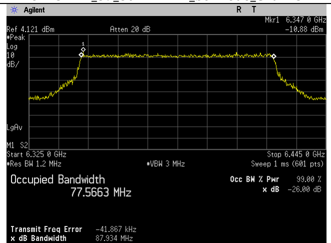
6385MHz_87_80MHz BW_be-mode_Chain 1
