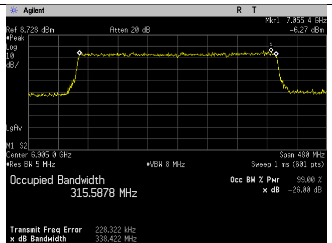
6905MHz_191_320MHz BW_be-mode_Chain 1
