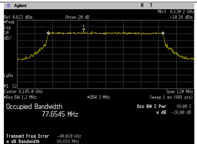
6145MHz_39_80MHz BW_be-mode_Chain 3
