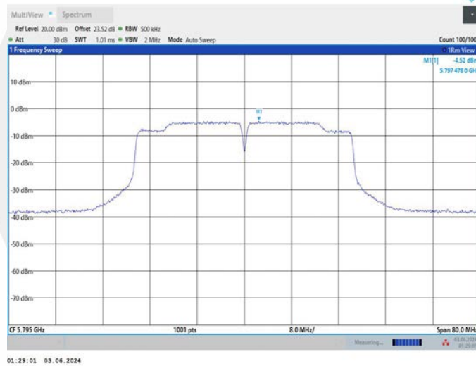
11N40MIMO_Ant2_5795
