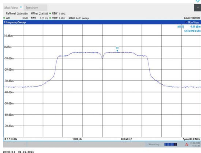
11N40MIMO_Ant1_5510
