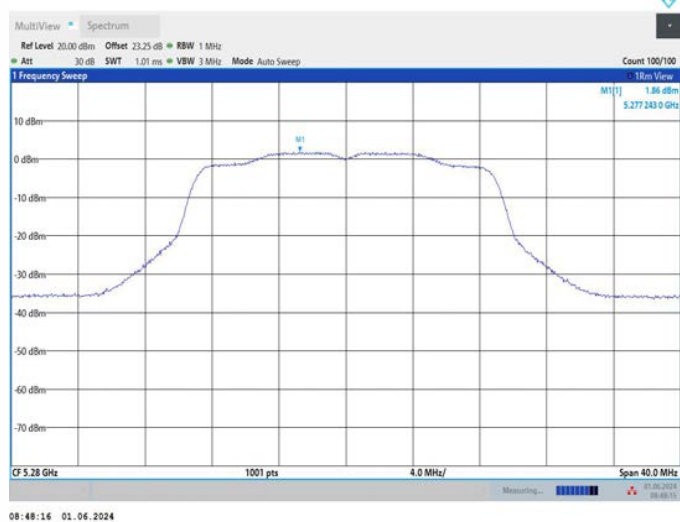
11N20MIMO_Ant1_5280
