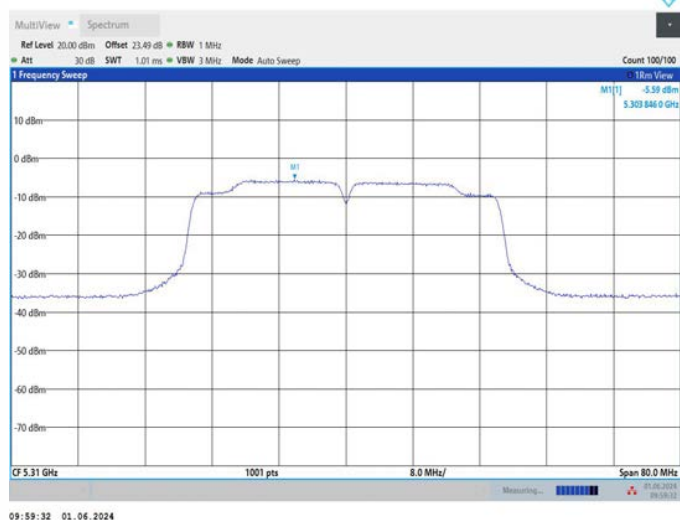
11N40MIMO_Ant2_5310
