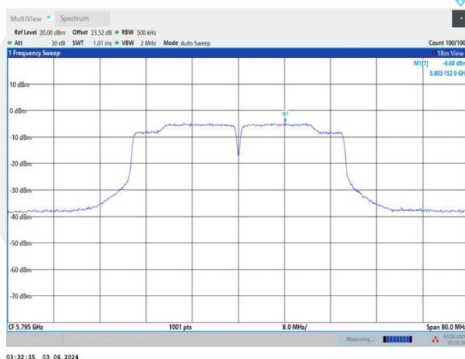
11AC40MIMO_Ant2_5795
