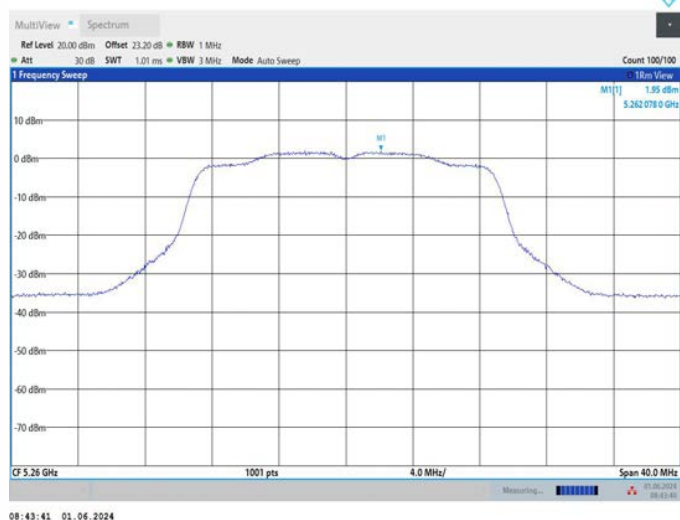
11N20MIMO_Ant2_5260
