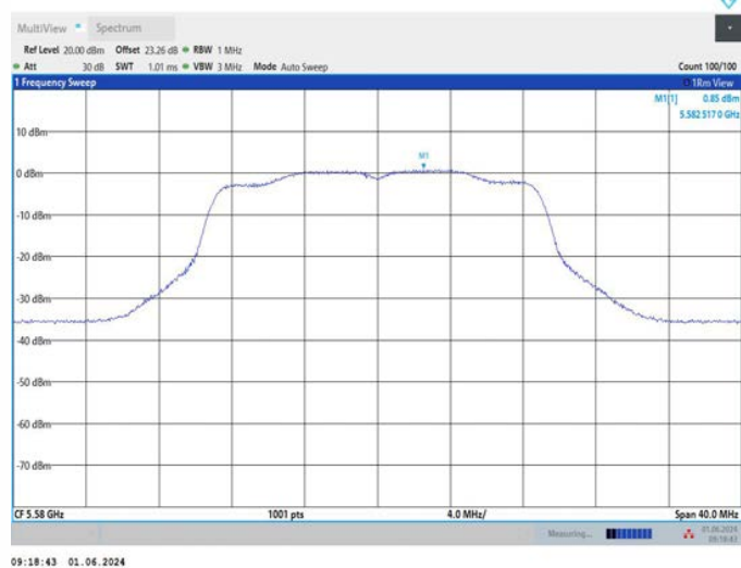
11N20MIMO_Ant1_5580
