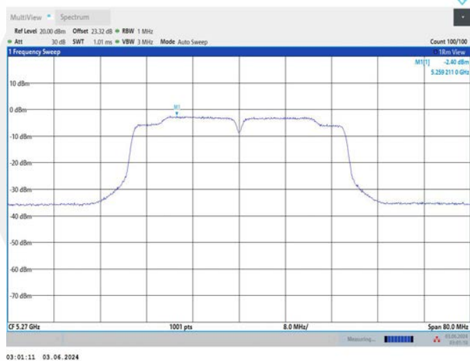
11AC40MIMO_Ant2_5270
