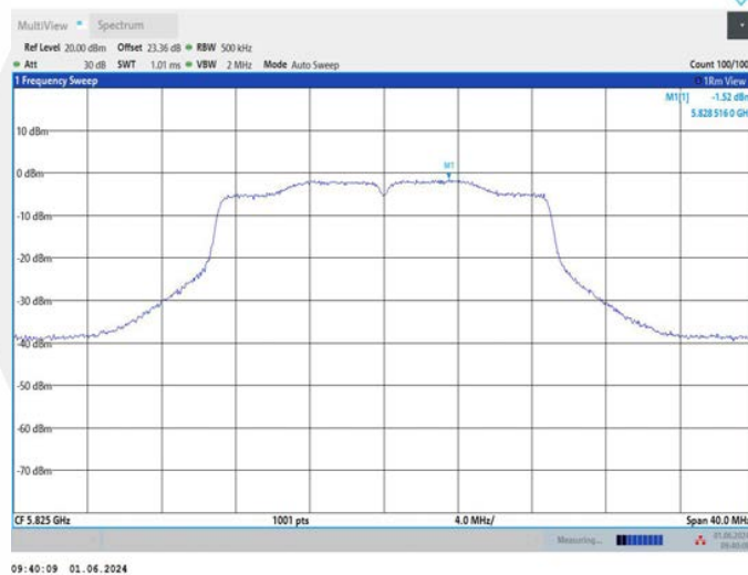
11N20MIMO_Ant2_5825
