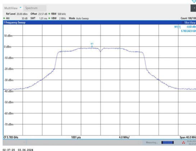
11AC20MIMO_Ant1_5785
