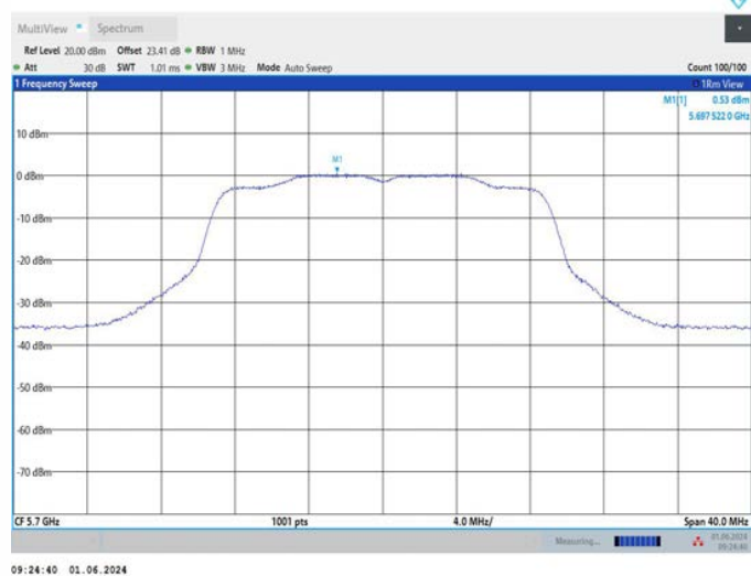
11N20MIMO_Ant2_5700
