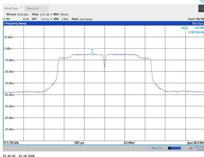
11AC40MIMO_Ant2_5795
