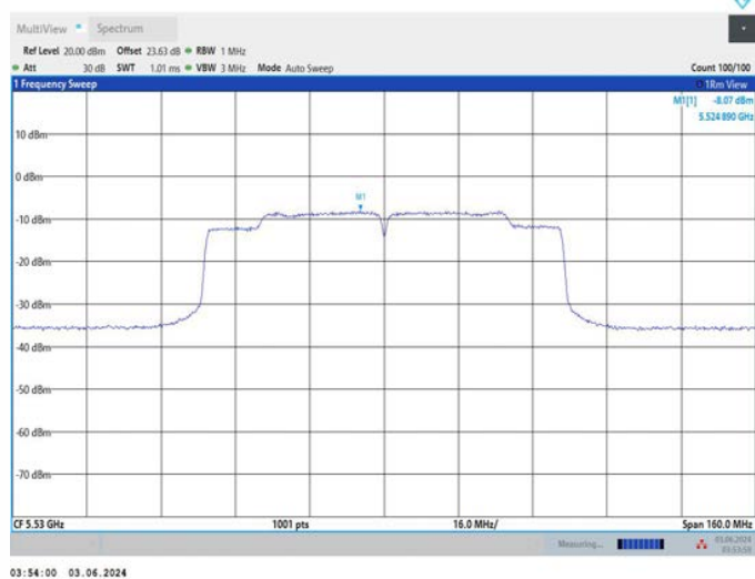
11AC80MIMO_Ant2_5530
