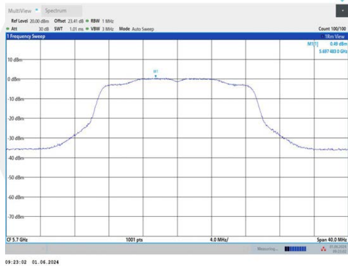
11N20MIMO_Ant2_5700
