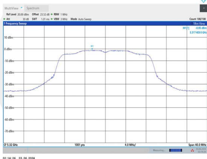
11AC20MIMO_Ant2_5320
