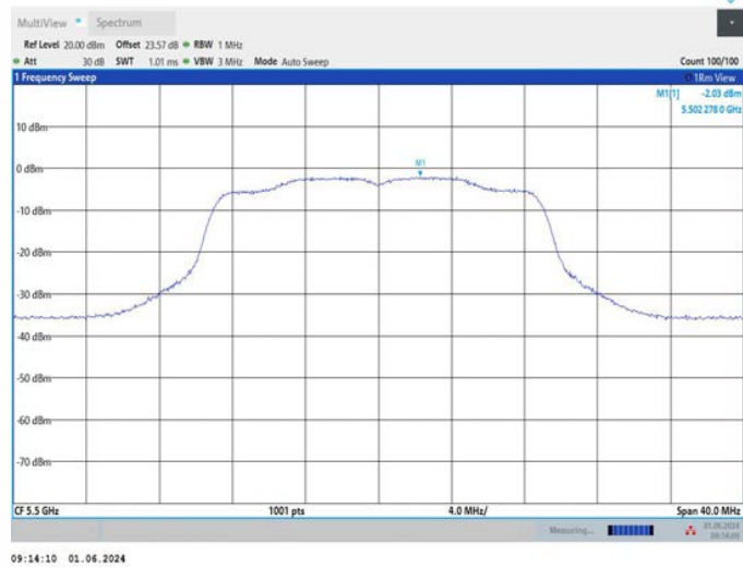
11N20MIMO_Ant2_5500
