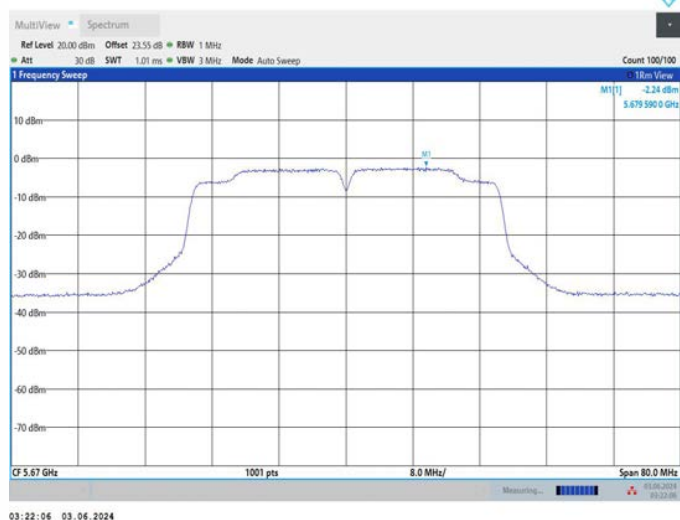
11AC40MIMO_Ant2_5670
