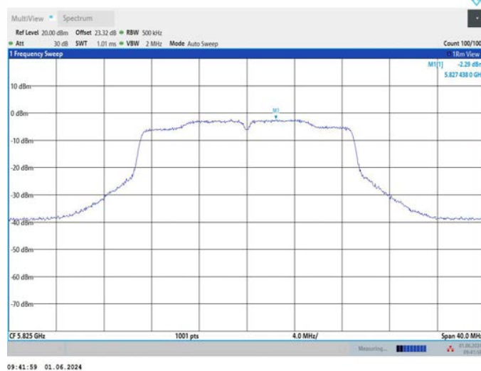
11N20MIMO_Ant2_5825
