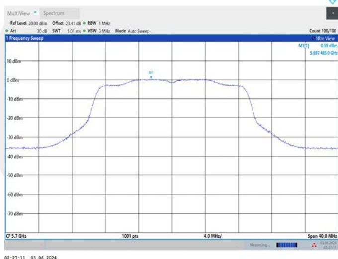
11AC20MIMO_Ant2_5700
