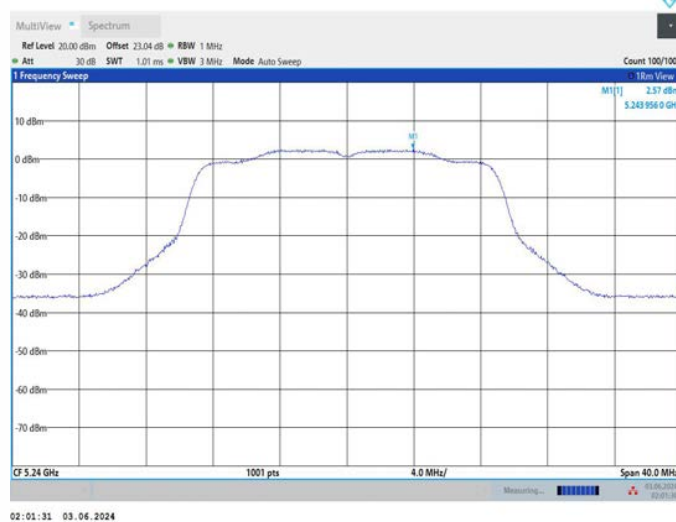
11AC20MIMO_Ant2_5240
