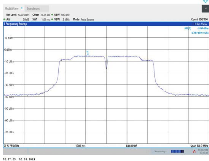
11AC40MIMO_Ant1_5755
