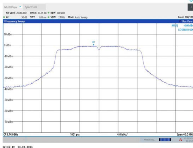
11AC20MIMO_Ant2_5745
