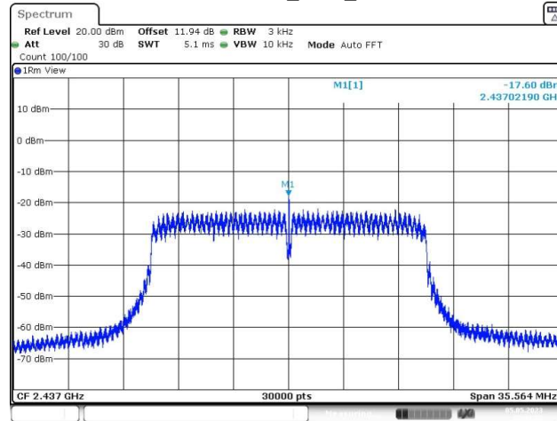
11N20SISO_Ant1_2437
