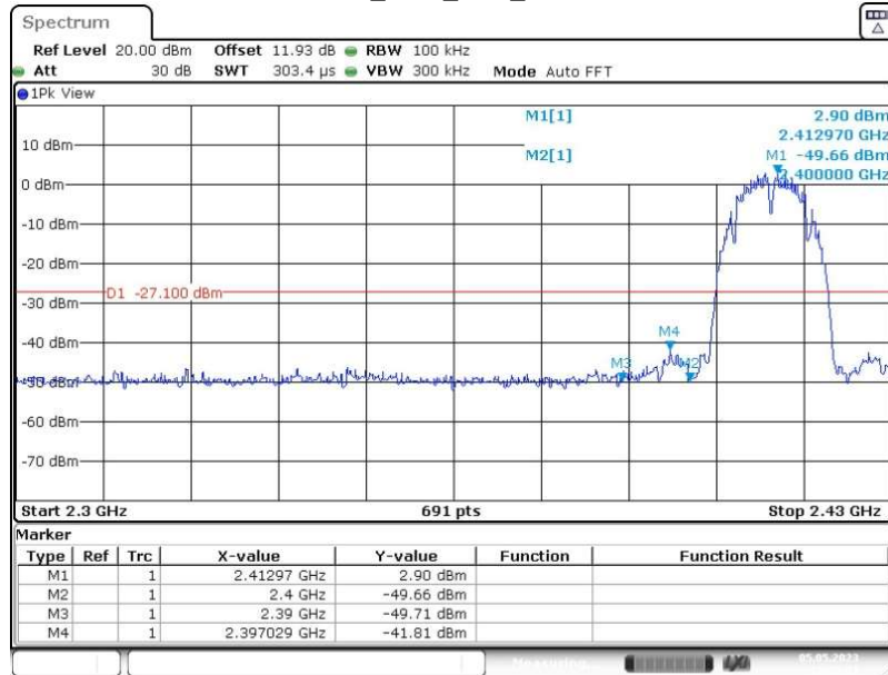
11B_Ant1_Low_2412
