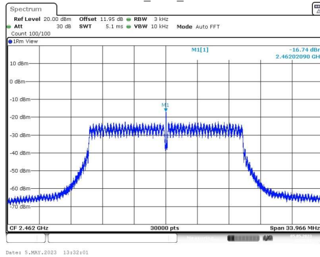
11G_Ant1_2462
