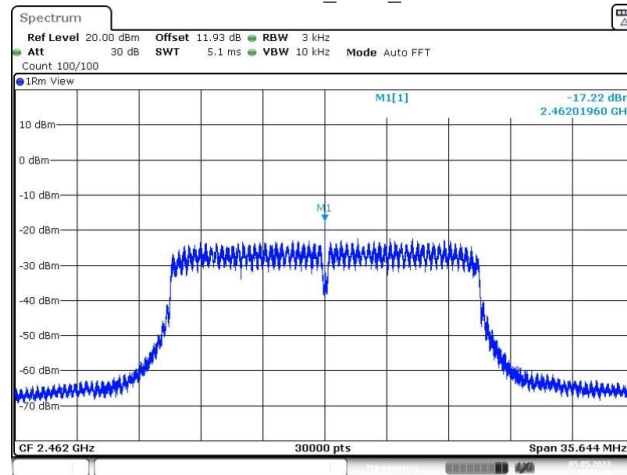
11N20SISO_Ant1_2462
