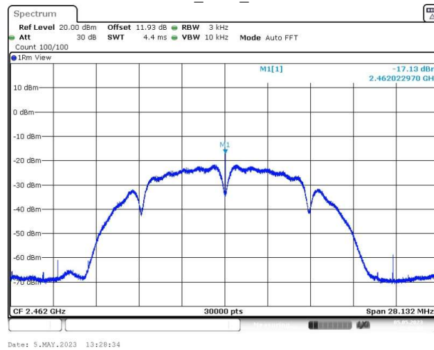
11B_Ant1_2462
