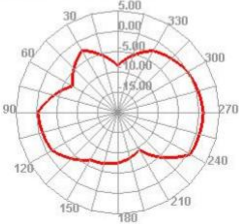
2500.000MHz E2
