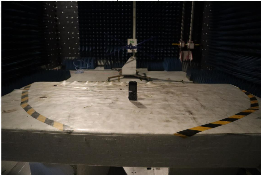
RE (Below 1GHz)
