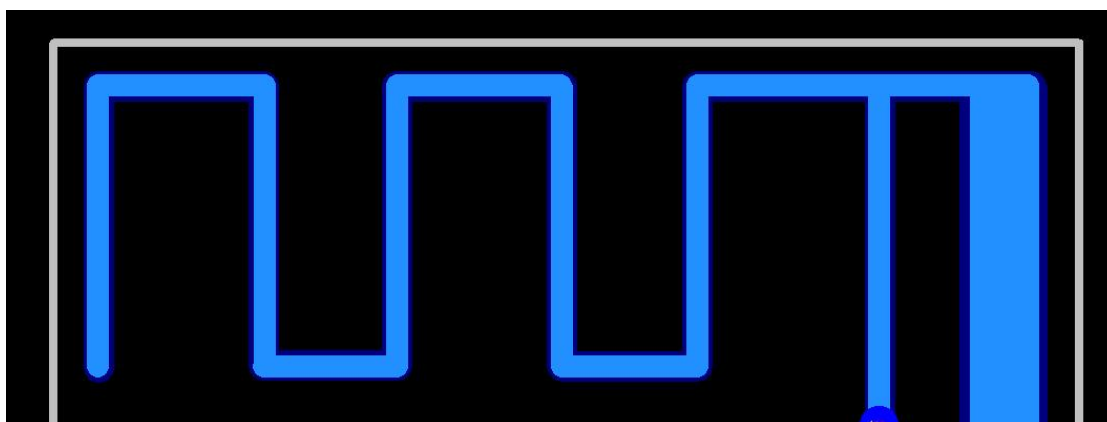
2.4G Antenna
