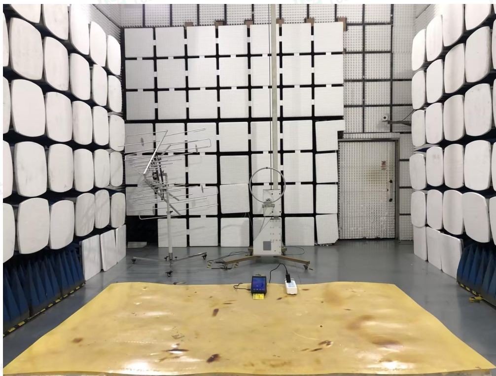
Fig. 1 (Below 30MHz)
