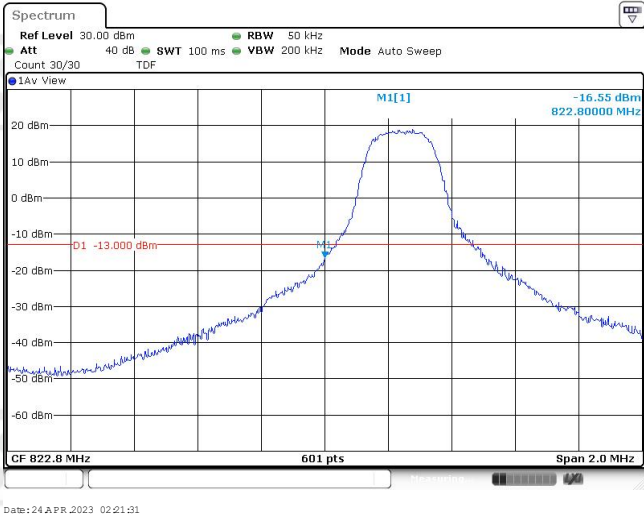
Band26-3MHz-QPSK-26793-1RB#14
