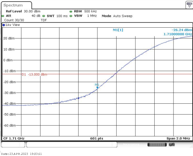
Band4-20MHz-QPSK-20050-1RB#99
