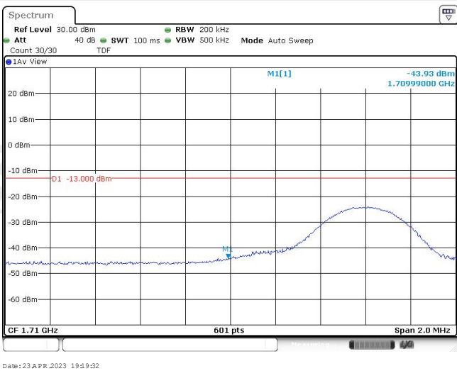
Band4-10MHz-QPSK-20000-50RB#0
