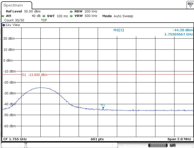
Band4-10MHz-QPSK-20350-1RB#0
