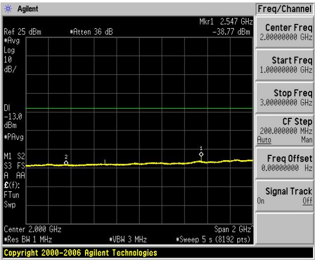
GPRS850-128-3000~10000MHz
