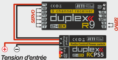
Fig. 5: Exemple de connexion avec RC Power Switch
