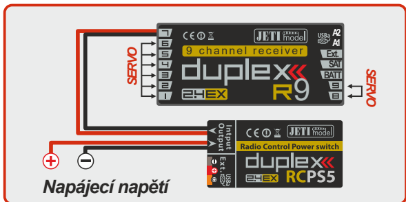
Obr. 5: Aplikační zapojení s RCPSwitchem
