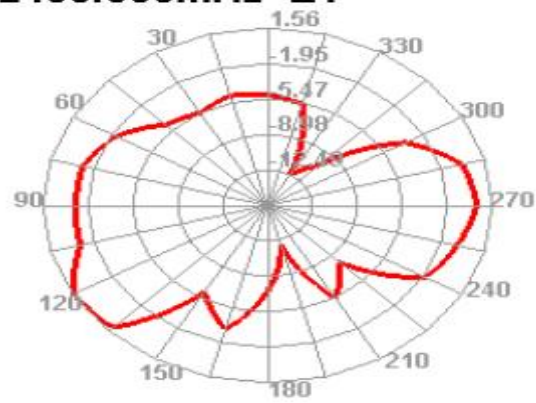
2400.000MHz E1
