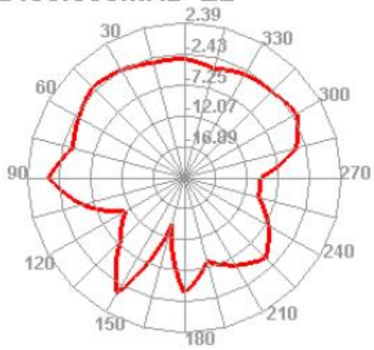
2450.000MHz E2
