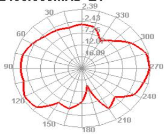
2450.000MHz E1
