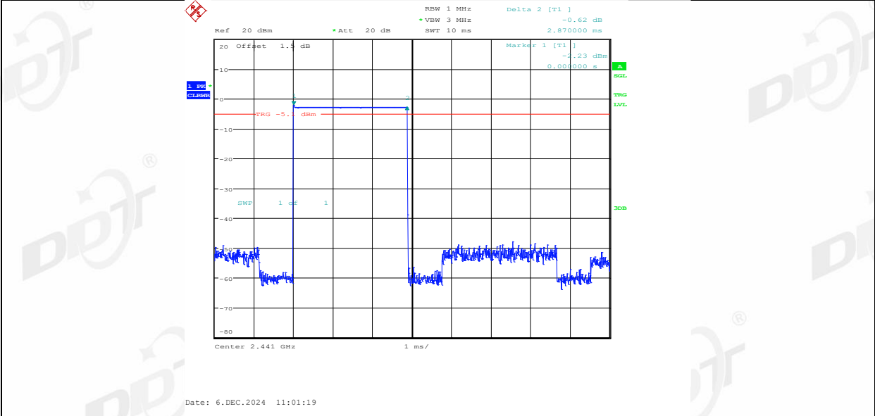
DH5_Ant1_Hop
