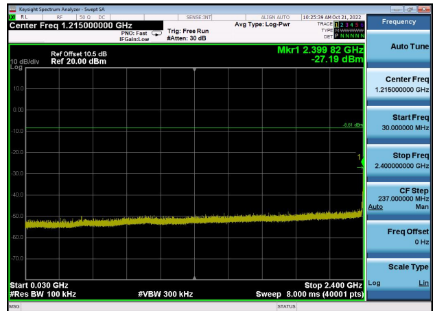
,Plot 3,30MHz~2400MHz-802.11b,2437MHz
