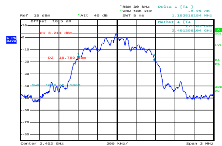
\pi/4 -DQPSK_Low
