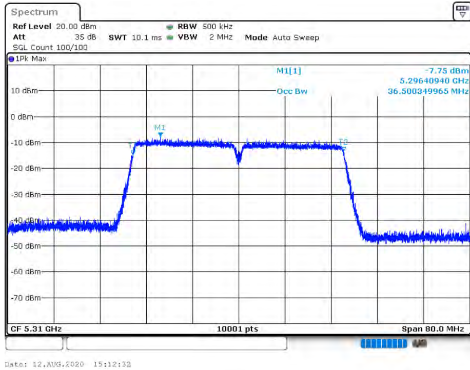
-26 dB BW NVNT 802.11n(HT40) 5310MHz Ant 2
