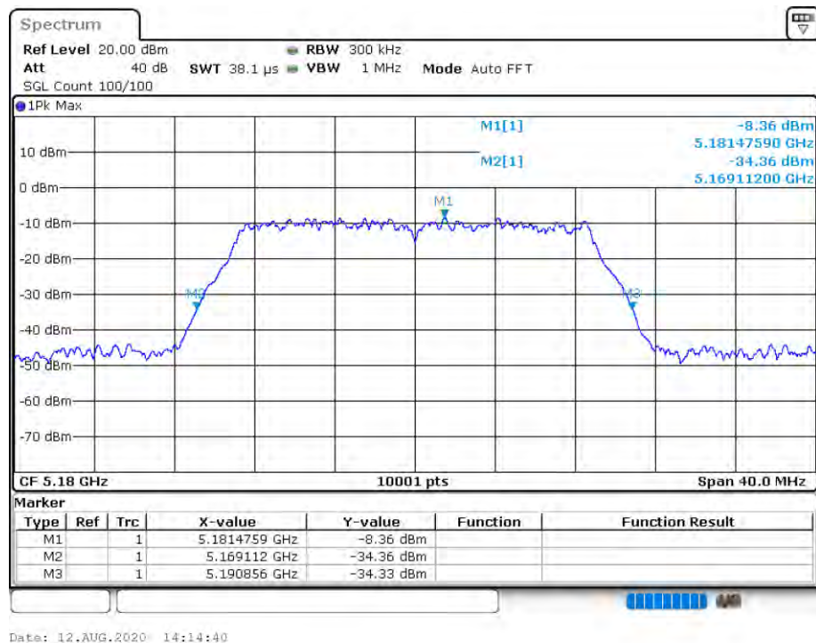
-26 dB BW NVNT 802.11ac20 5180MHz Ant 2
