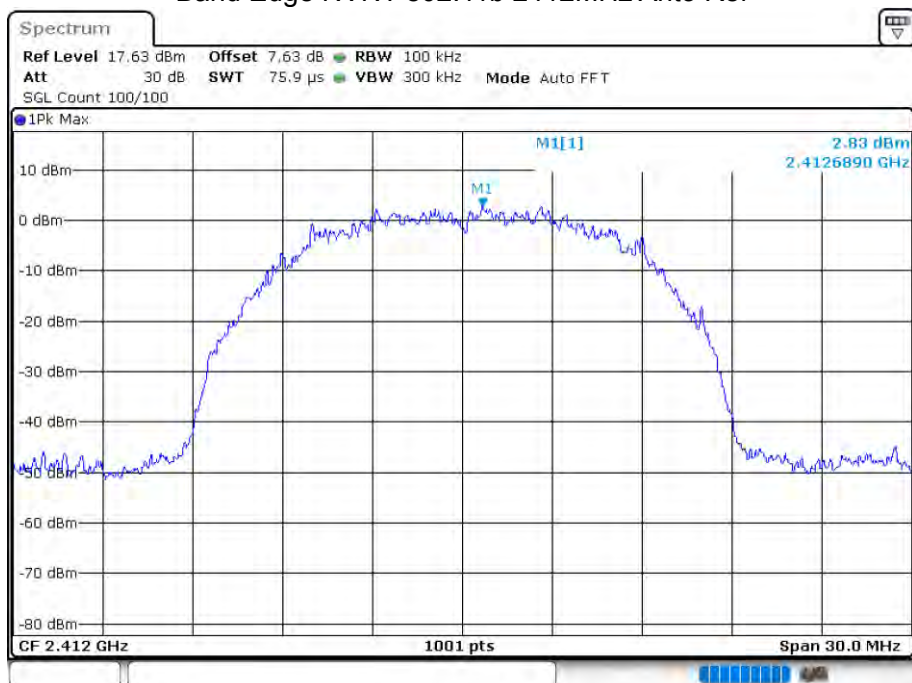
Band Edge NVNT 802.11b 2412MHz Ant3 Ref
