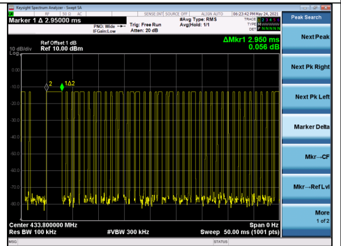
Ton 3 time
