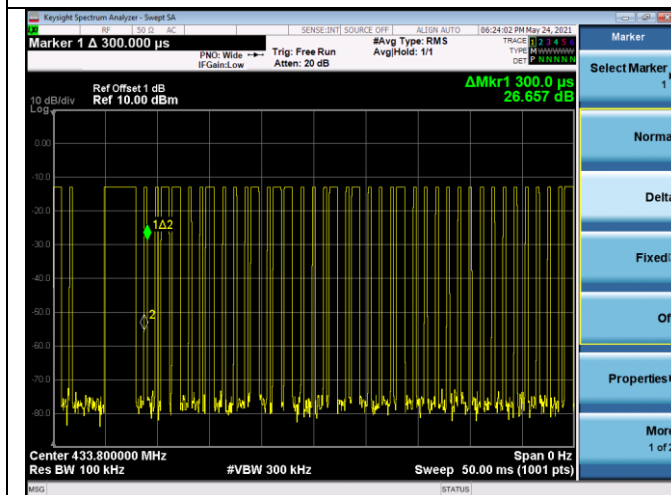
Ton 2 time
