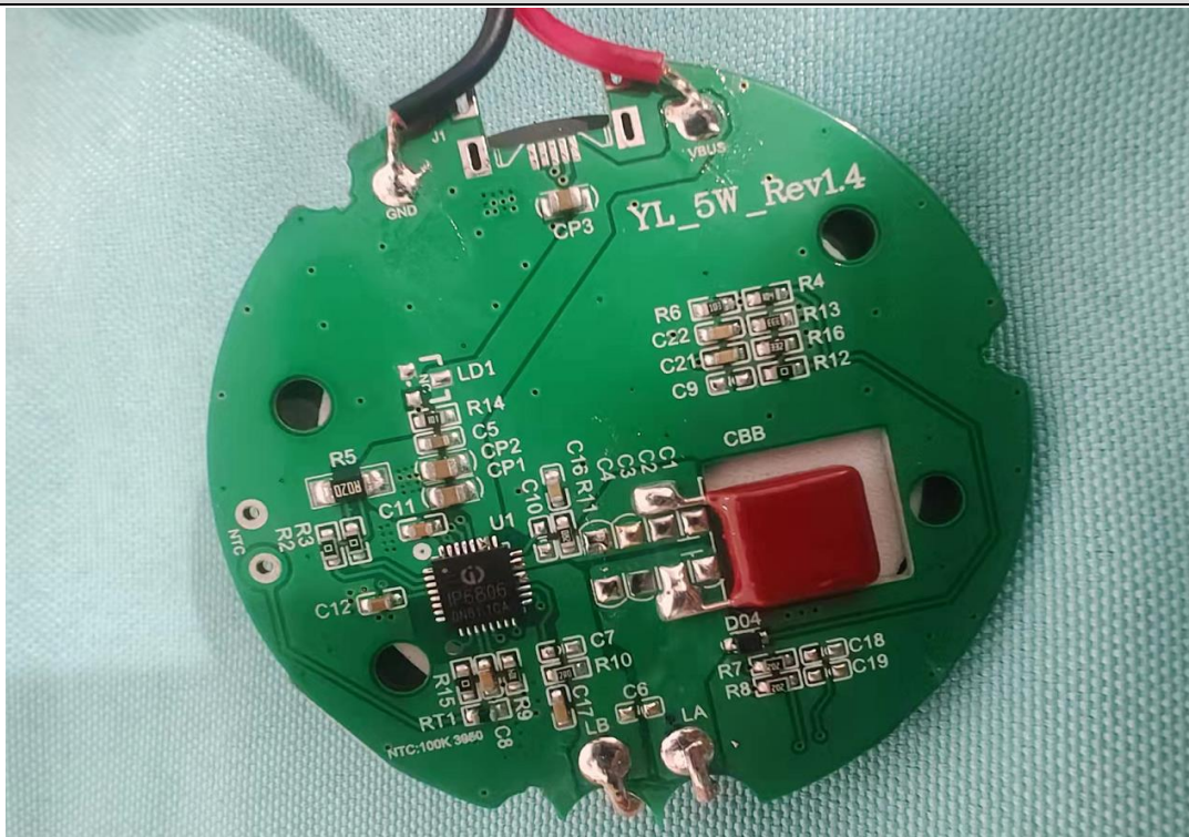
EUT Photo
