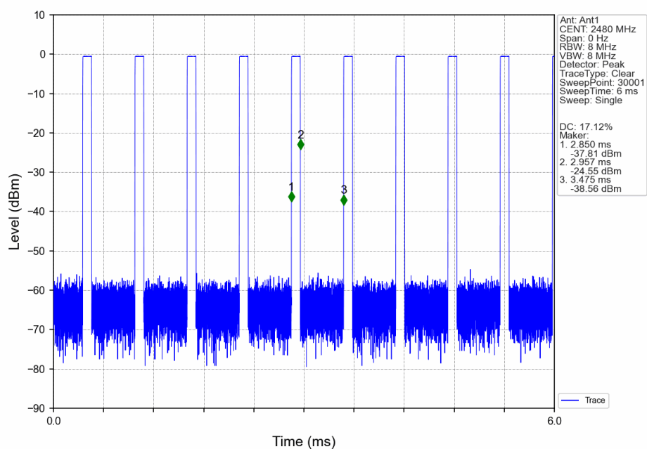
GFSK_HCH_2480MHz_Ant1_NTNV
