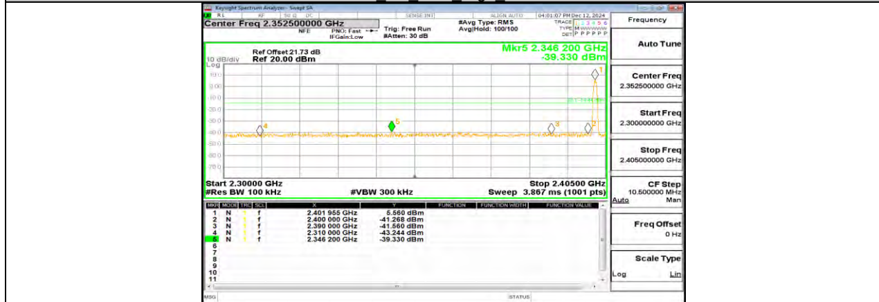
BLE 125K Ant1 Low 2402
