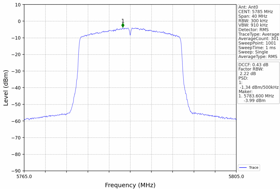
802.11ax(HEW20)_MCH_5785MHz_RU242_Left_Ant0_NTNV
