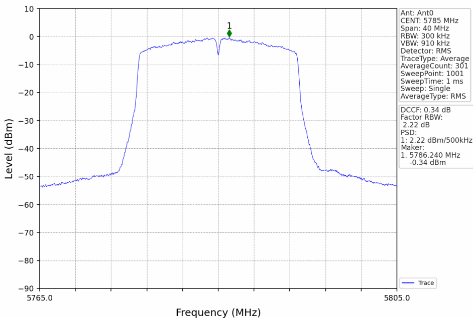
802.11n(HT20)_MCH_5785MHz_Ant0_NTNV
