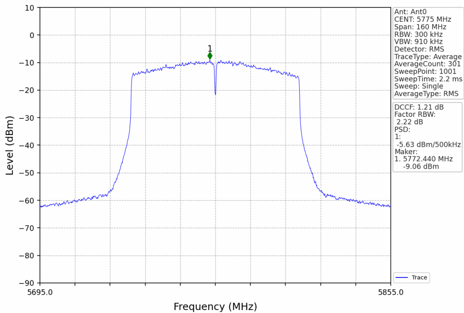
802.11ac(VHT80)_MCH_5775MHz_Ant0_NTNV
