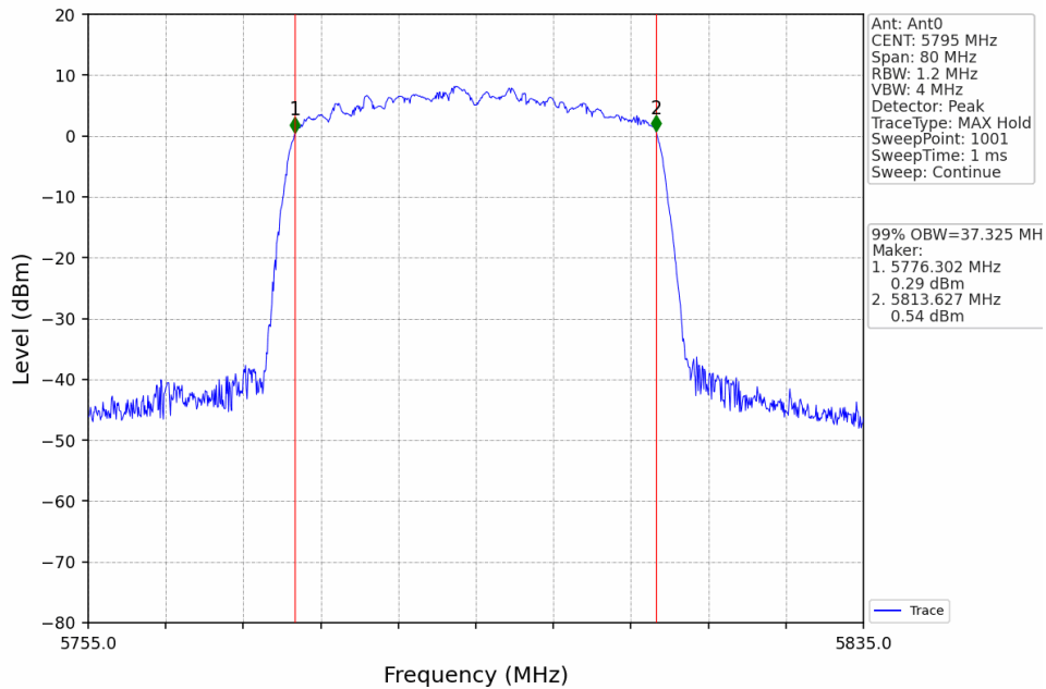
802.11ax(HEW40)_HCH_5795MHz_RU484_Left_Ant0_NTNV
