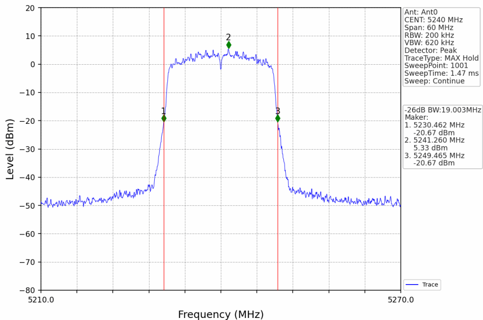
802.11n(HT20)_HCH_5240MHz_Ant0_NTNV
