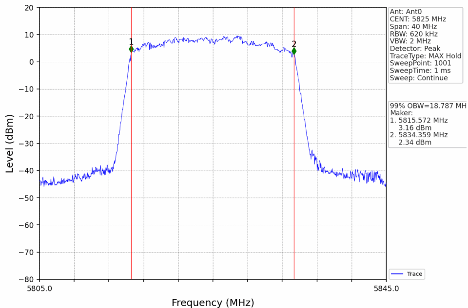
802.11ax(HEW20)_HCH_5825MHz_RU242_Left_Ant0_NTNV
