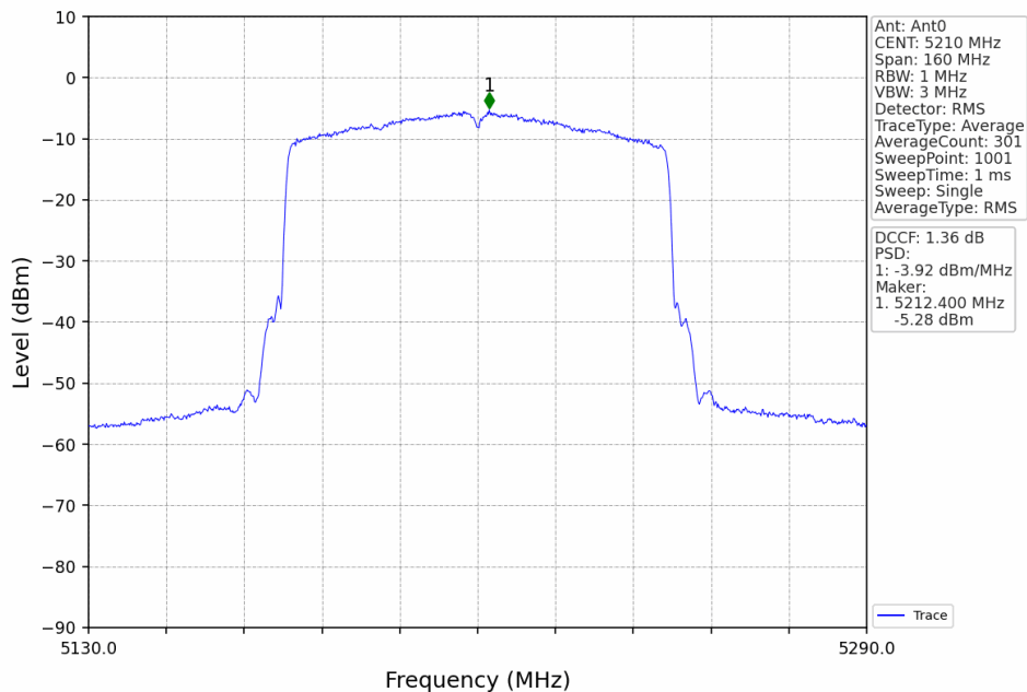
802.11ax(HEW80)_MCH_5210MHz_RU996_Left_Ant0_NTNV
