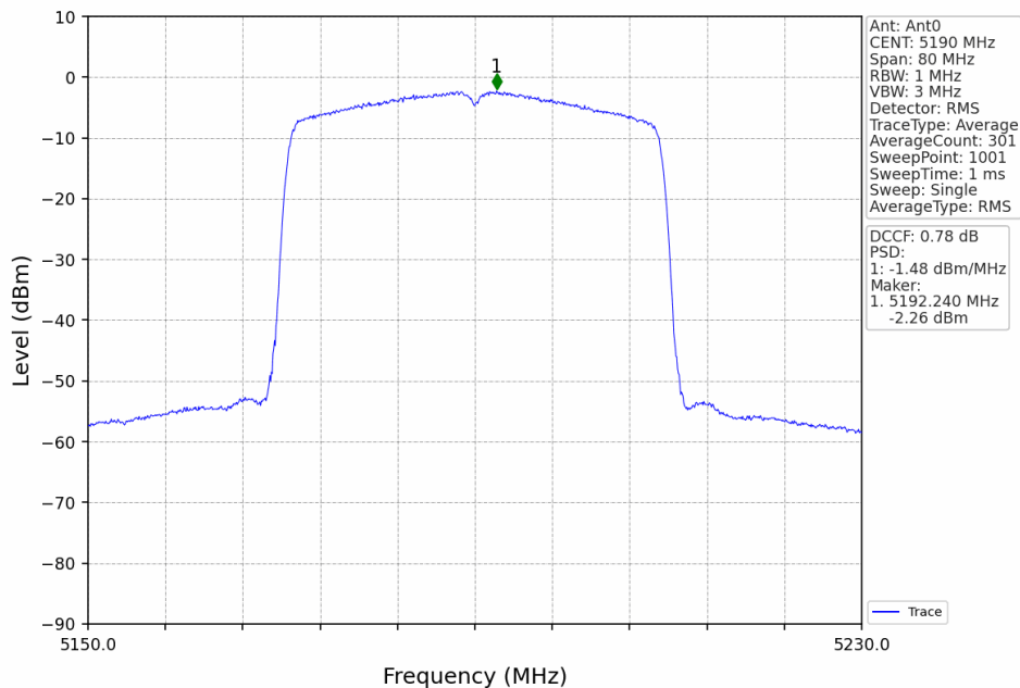
802.11ax(HEW40)_LCH_5190MHz_RU484_Left_Ant0_NTNV
