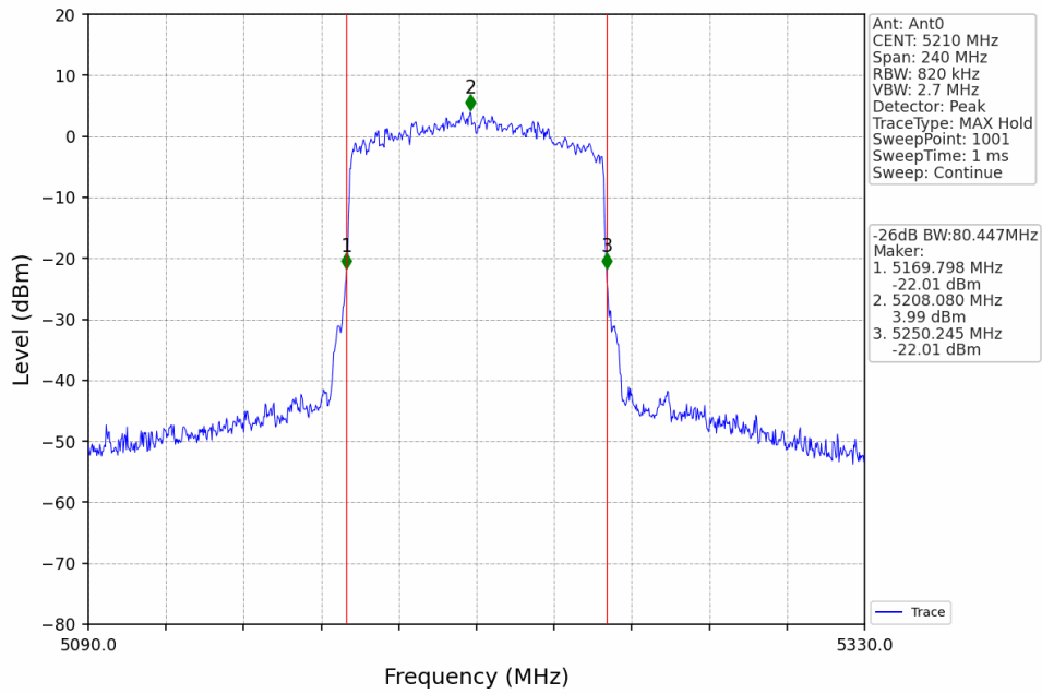
802.11ax(HEW80)_MCH_5210MHz_RU996_Left_Ant0_NTNV
