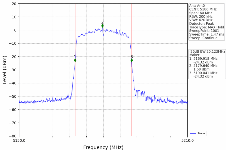
802.11ax(HEW20)_LCH_5180MHz_RU242_Left_Ant0_NTNV
