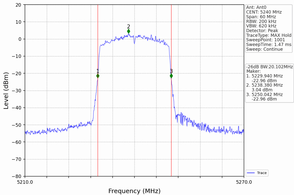
802.11ax(HEW20)_HCH_5240MHz_RU242_Left_Ant0_NTNV
