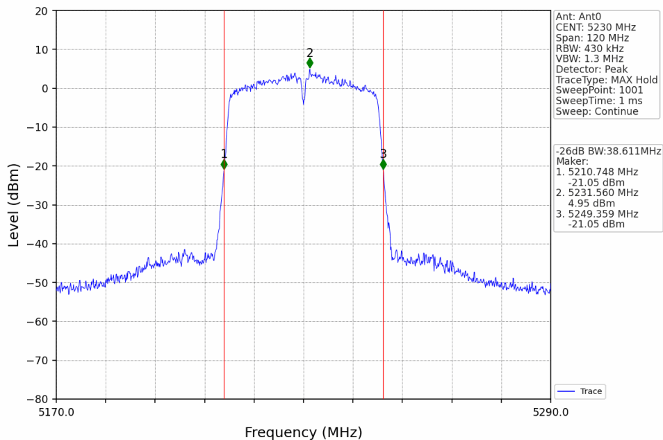
802.11n(HT40)_HCH_5230MHz_Ant0_NTNV
