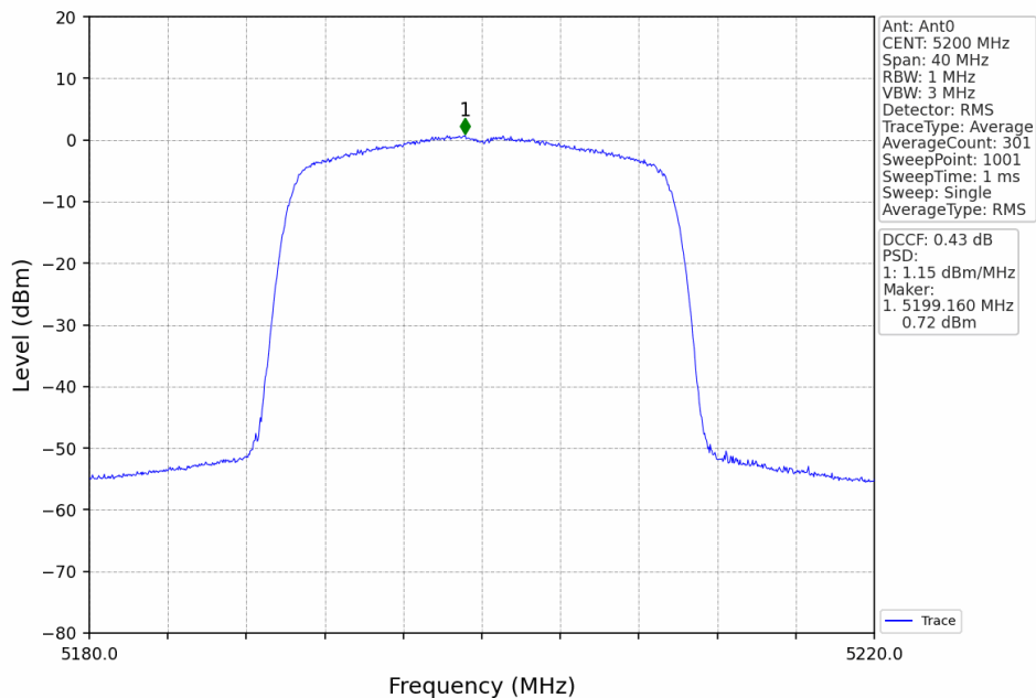
802.11ax(HEW20)_MCH_5200MHz_RU242_Left_Ant0_NTNV
