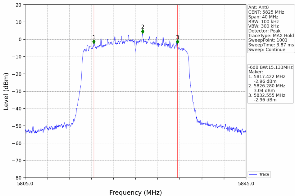
802.11ax(HEW20)_HCH_5825MHz_RU242_Left_Ant0_NTNV
