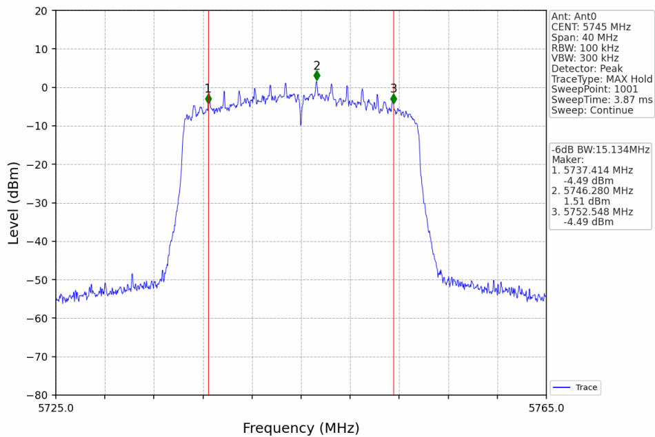
802.11ax(HEW20)_LCH_5745MHz_RU242_Left_Ant0_NTNV
