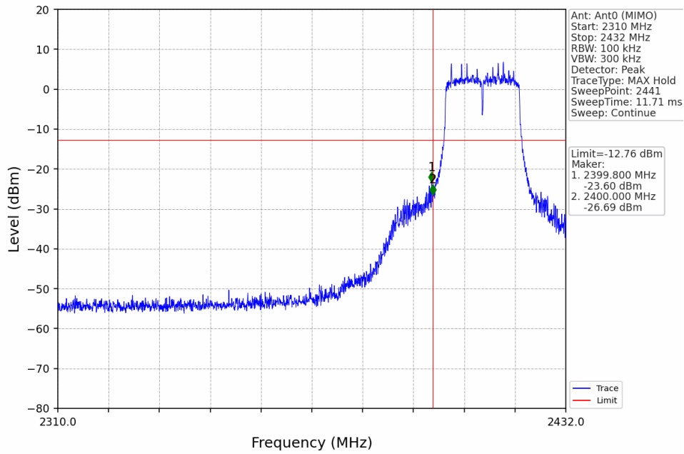
802.11n(HT20)_LCH_2412MHz_Ant0 (MIMO)_NTNV
