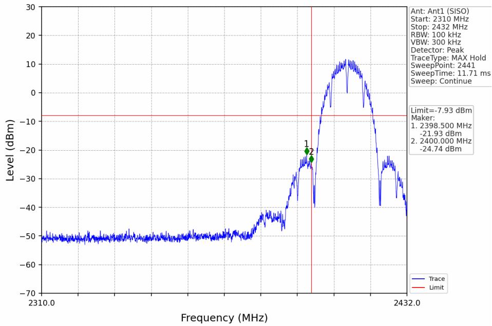
802.11b_LCH_2412MHz_Ant1 (SISO)_NTNV
