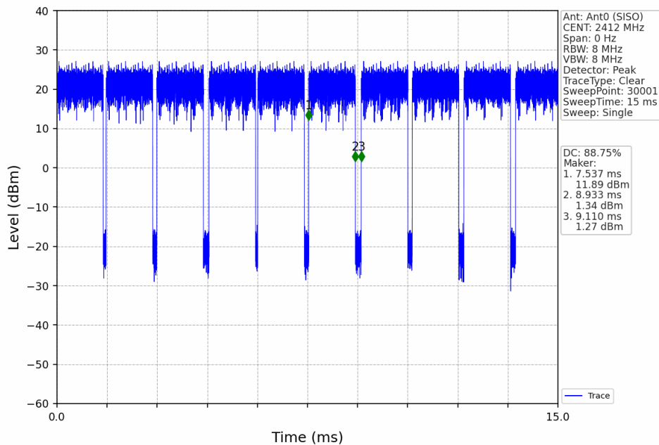
802.11g_LCH_2412MHz_Ant0 (SISO)_NTNV
