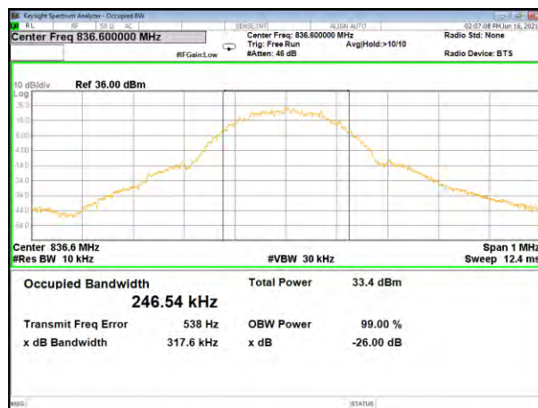
EGPRS850_Middle
