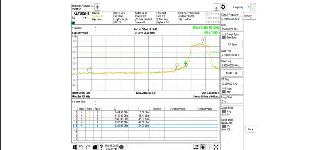
11G_Ant1_Low_2412
