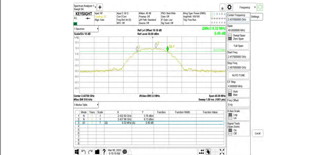
11B_Ant1_2437
