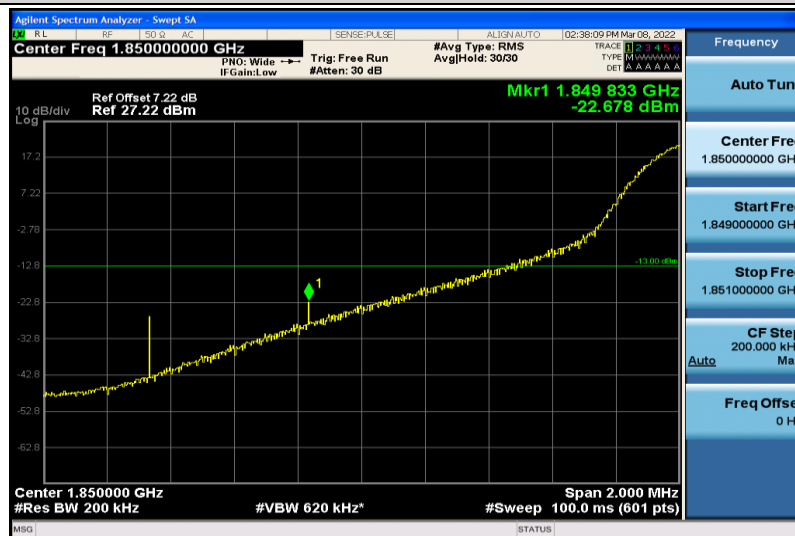
Band2-20MHz-64QAM-18700-1RB#0
