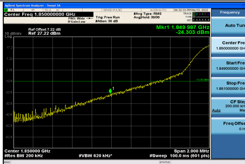
Band2-20MHz-16QAM-18700-1RB#0
