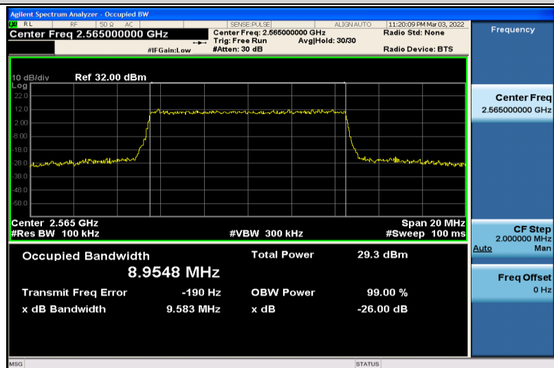
Band7-10MHz-QPSK-21400-50RB#0-8.9548
