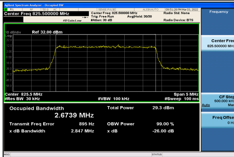
Band5-3MHz-QPSK-20415-15RB#0-2.6739
