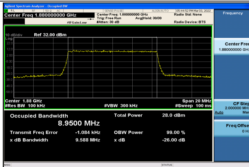
Band2-10MHz-16QAM-18900-50RB#0-8.9500
