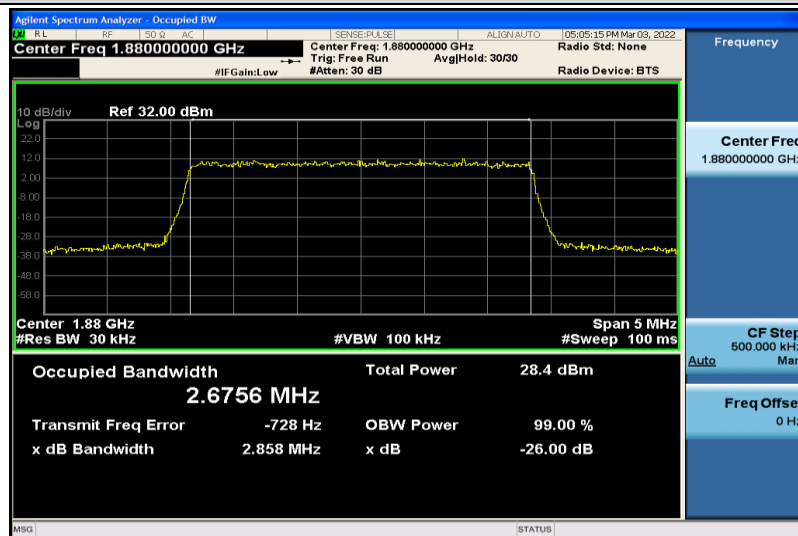
Band2-3MHz-QPSK-18900-15RB#0-2.6756
