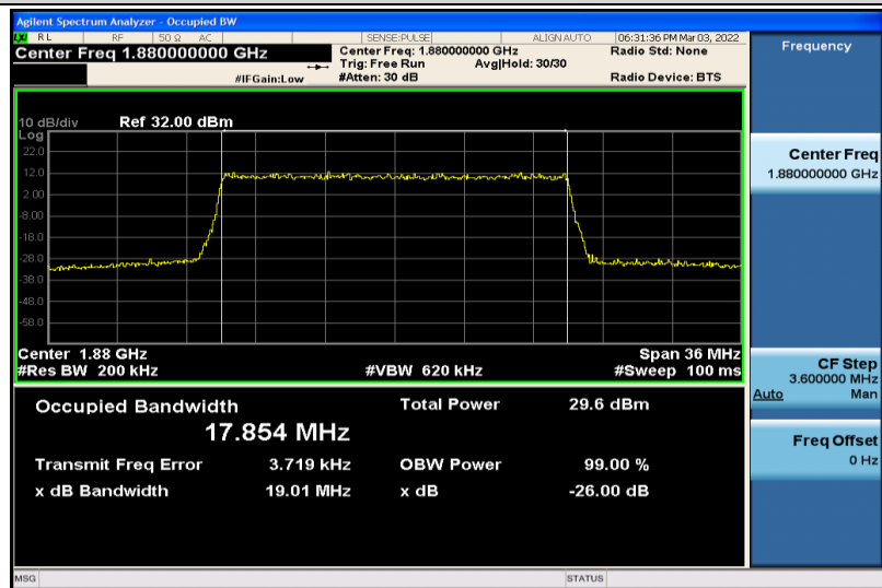
Band2-20MHz-QPSK-18900-100RB#0-17.854
