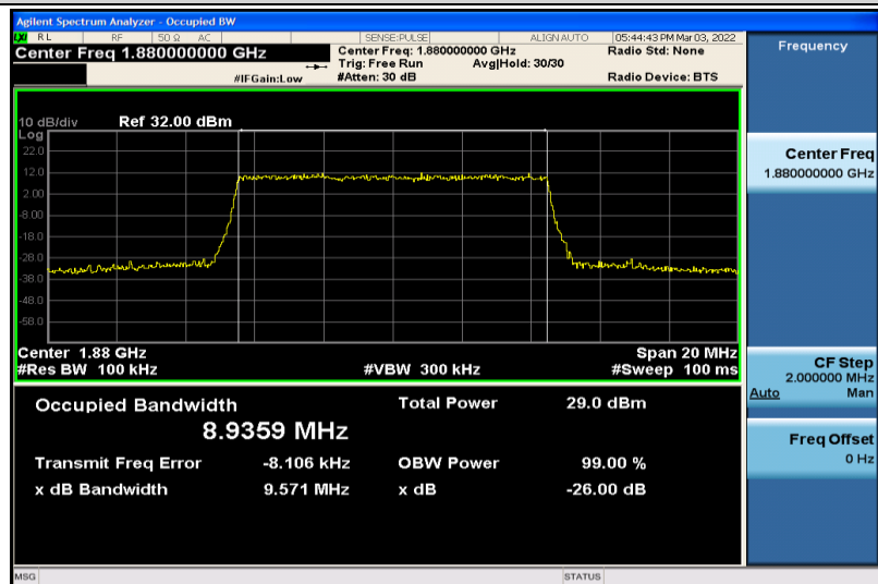
Band2-10MHz-QPSK-18900-50RB#0-8.9359
