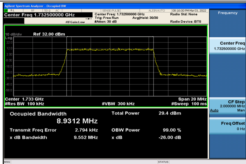
Band4-10MHz-QPSK-20175-50RB#0-8.9312
