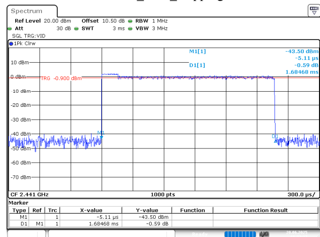
2EDR_DH3_Hopping
