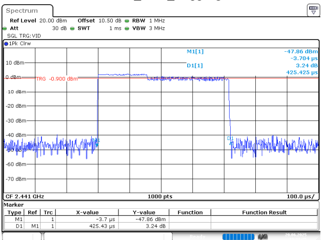
2EDR_DH1_Hopping
