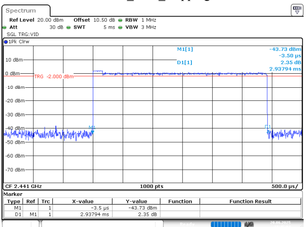
2EDR_DH5_Hopping
