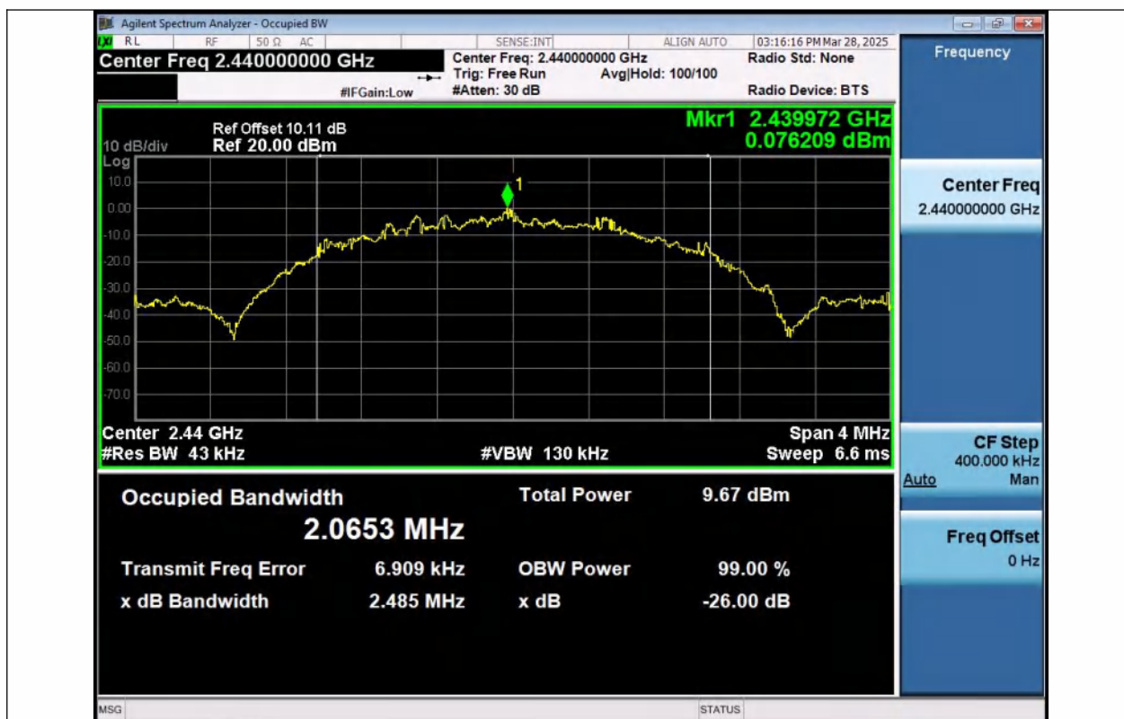
BLE 2M-Ant1-2440
