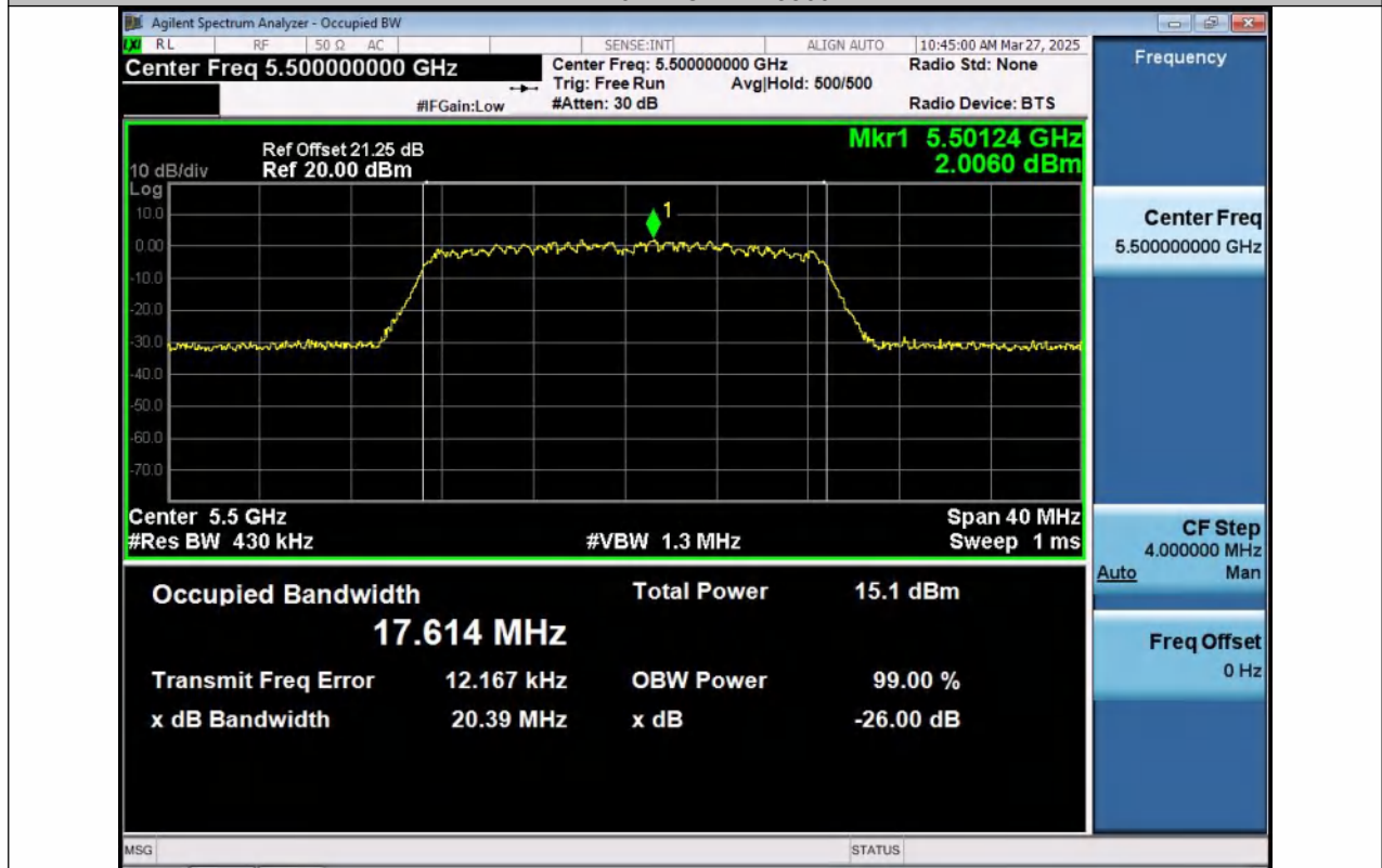
11N20MIMO-Ant2-5500
