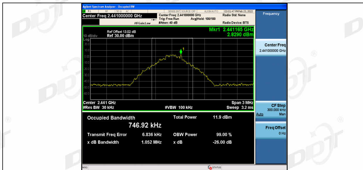
DH5 Ant1 2480
