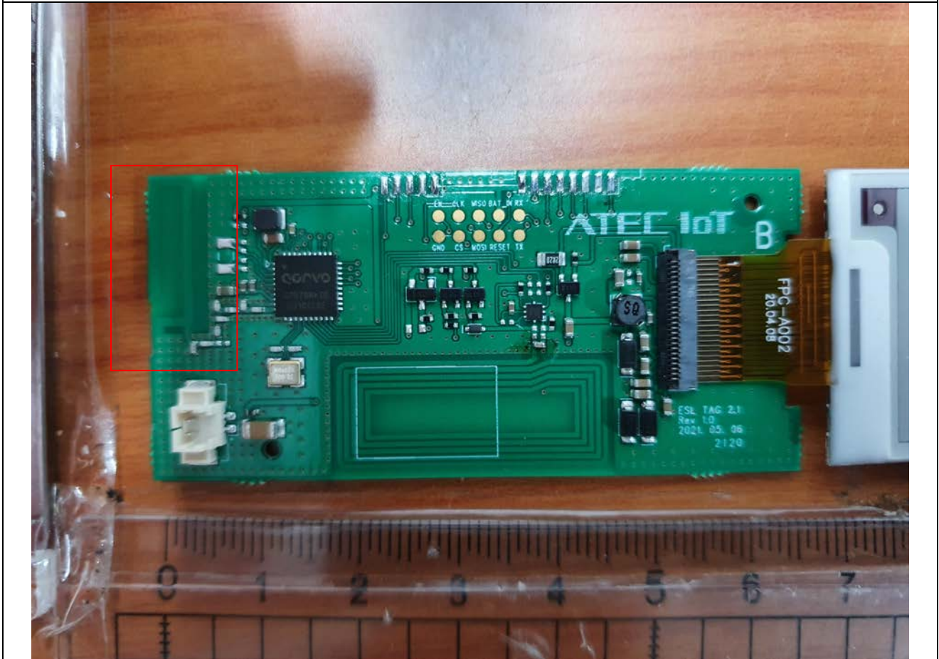
ANTENNA(2.4 GHz)
