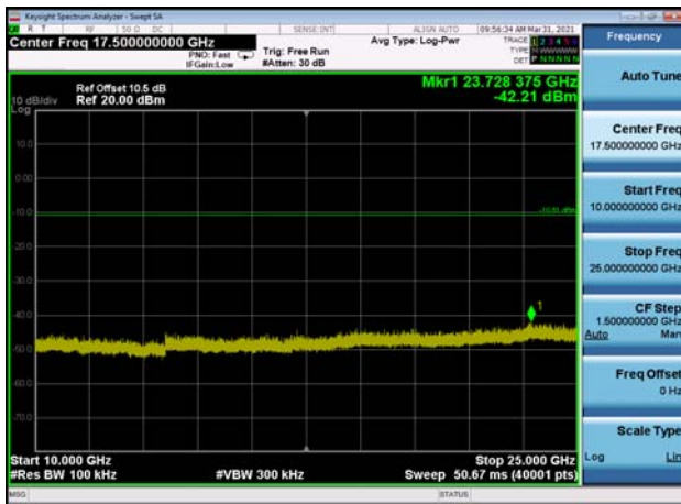
,Plot 5,10000MHz~25000MHz-802.11b ,2462MHz,Ant1
