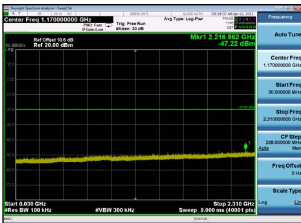
,Plot 3,30MHz~2310MHz-802.11ax(HE20) ,2462MHz,Ant0
