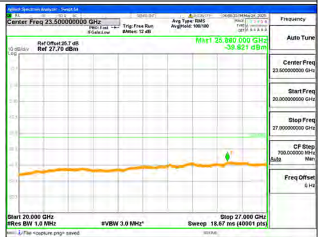
B41-20G-27G / 15MHz / Mid CH / QPSK
