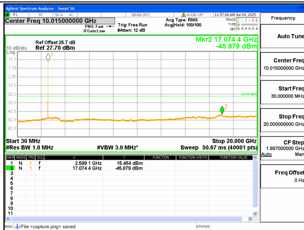
41C-30M-20G / 20+5MHz / QPSK / Mid CH / 1@99-1@0
