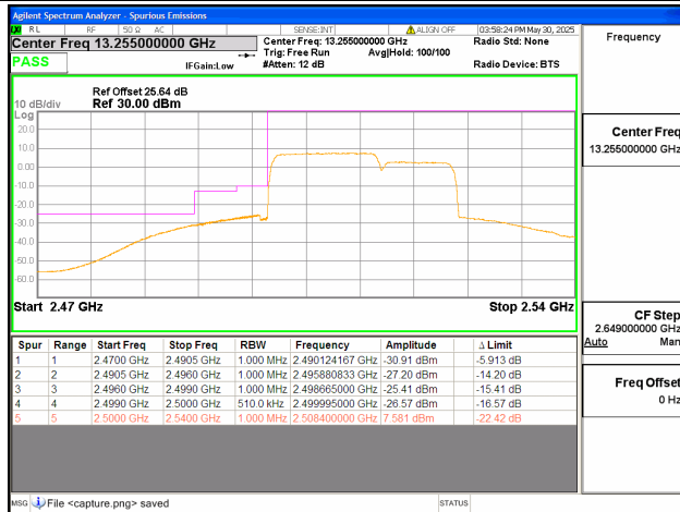
7C / 15+10MHz / Low CH / QPSK / 75#0-50#0
