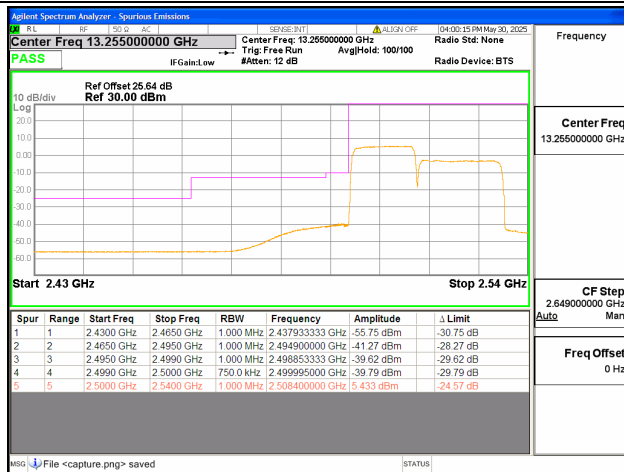
7C / 15+20MHz / Low CH / QPSK / 75#0-100#0
