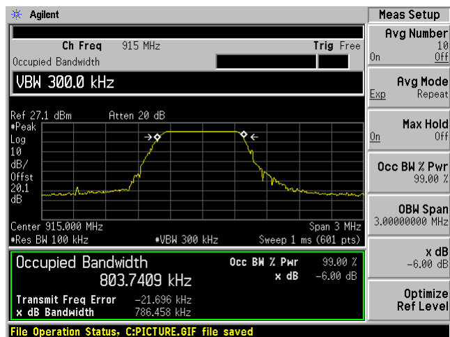
6 dB OBW
