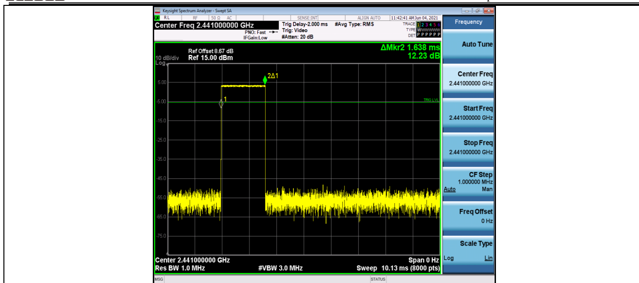
DH3_Ant1_Hop_2441
