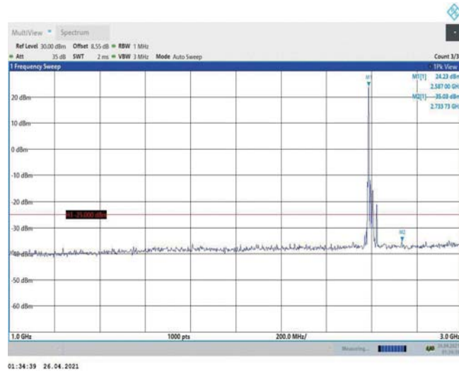
Band38-20MHz-QPSK-38000-1RB#0-Range2:1000~3000MHz
