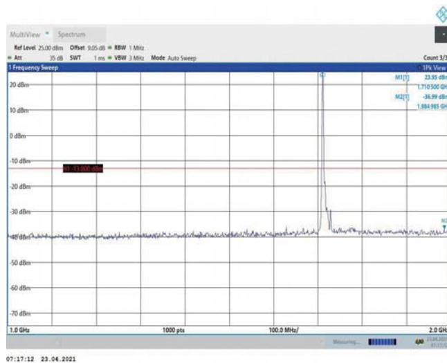
Band4-10MHz-QPSK-20000-1RB#0-Range2:1000~2000MHz
