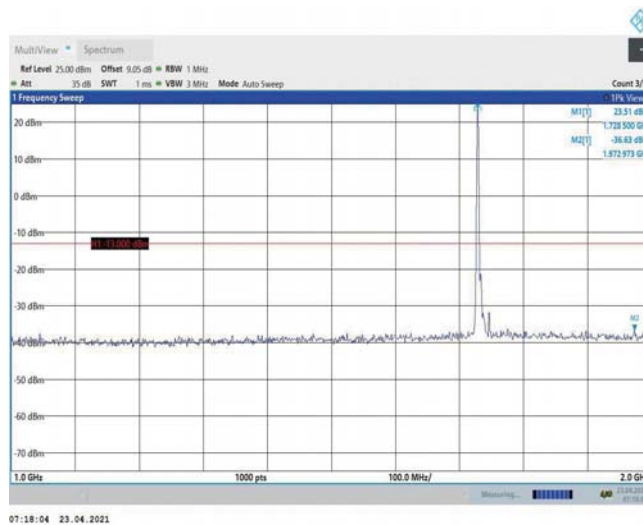
Band4-10MHz-QPSK-20175-1RB#0-Range2:1000~2000MHz
