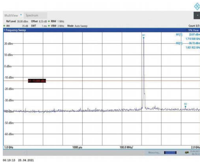
Band4-3MHz-16QAM-19965-1RB#0-Range2:1000~2000MHz
