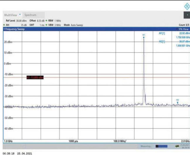
Band4-5MHz-QPSK-20375-1RB#0-Range2:1000~2000MHz
