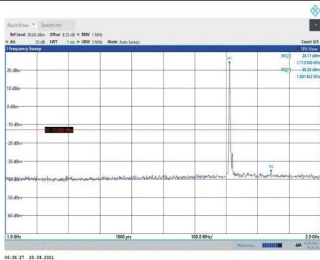
Band4-5MHz-QPSK-19975-1RB#0-Range2:1000~2000MHz
