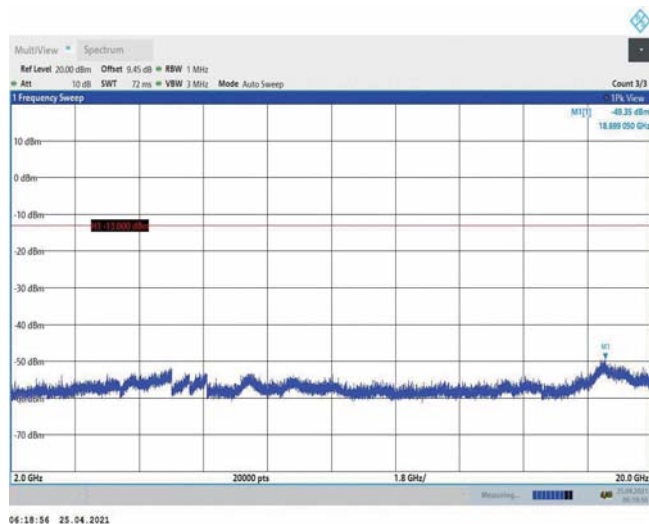
Band4-3MHz-QPSK-19965-1RB#0-Range3:2000~20000MHz
