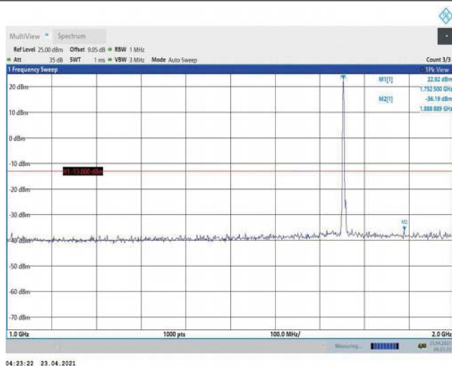
Band4-3MHz-QPSK-20385-1RB#0-Range2:1000~2000MHz
