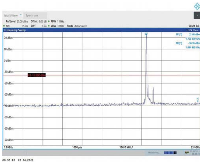
Band4-20MHz-QPSK-20175-1RB#0-Range2:1000~2000MHz
