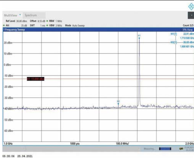
Band4-1.4MHz-QPSK-19957-1RB#0-Range2:1000~2000MHz
