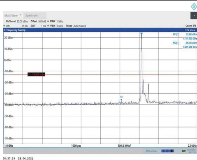
Band4-20MHz-QPSK-20050-1RB#0-Range2:1000~2000MHz
