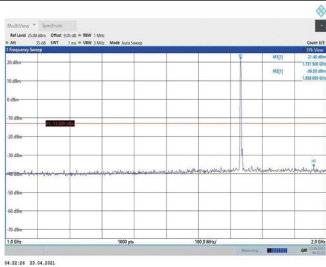
Band4-3MHz-QPSK-20175-1RB#0-Range2:1000~2000MHz
