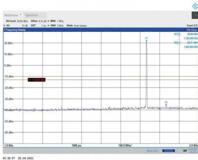
Band4-1.4MHz-QPSK-20175-1RB#0-Range2:1000~2000MHz
