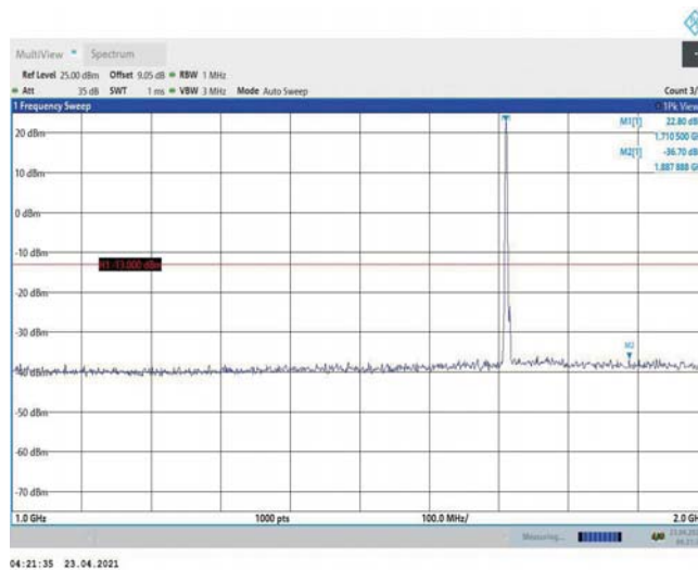
Band4-3MHz-QPSK-19965-1RB#0-Range2:1000~2000MHz
