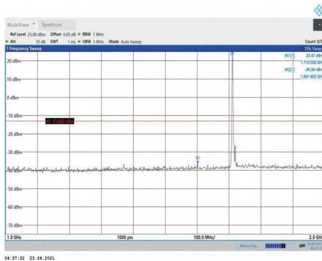
Band4-5MHz-QPSK-19975-1RB#0-Range2:1000~2000MHz
