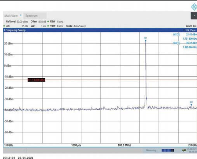
Band4-3MHz-QPSK-20175-1RB#0-Range2:1000~2000MHz
