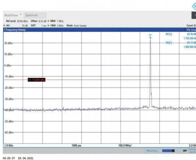
Band4-3MHz-QPSK-20385-1RB#0-Range2:1000~2000MHz
