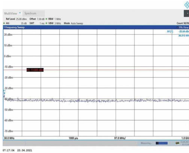
Band4-10MHz-QPSK-20000-1RB#0-Range1:30~1000MHz
